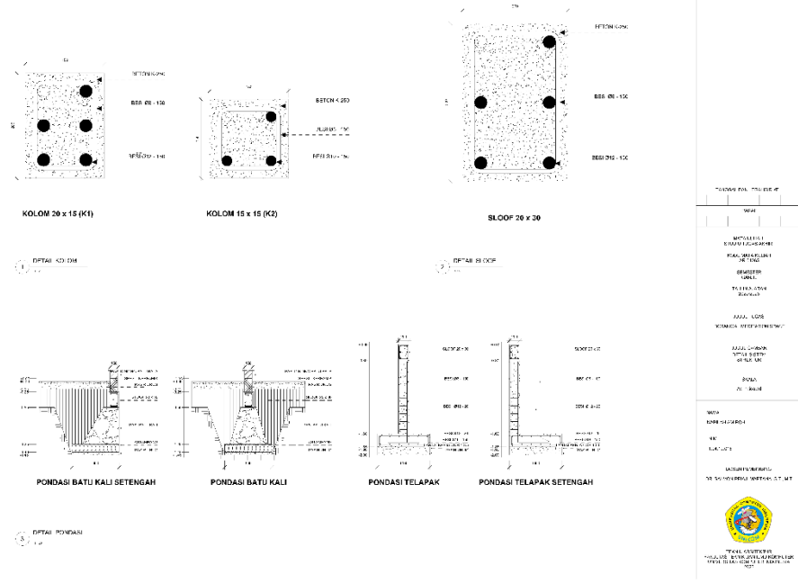
Gambar 6.15 Detail Pondasi (Dokumentasi Pribadi, 2023)
