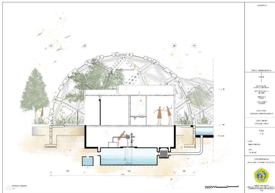
Gambar 6.9 Potongan Prinsip (Dokumentasi Pribadi, 2023)
