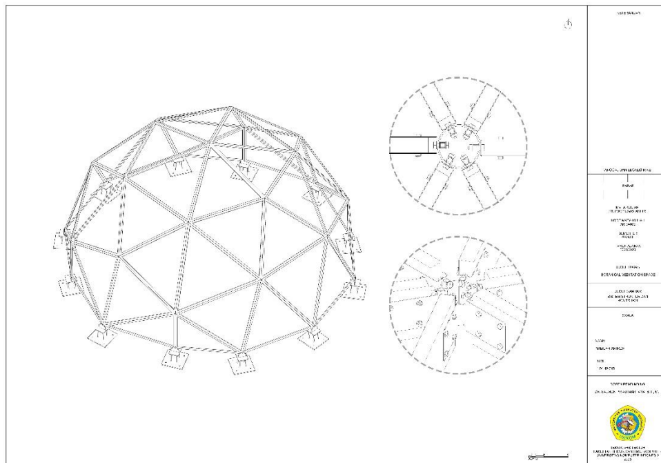
Gambar 6.16 Detail Struktur Dome (Dokumentasi Pribadi, 2023)
