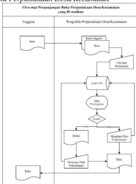
Gambar 5 Flow Map Perpanjangan Buku Perpustakaan Desa/Kecamatan
