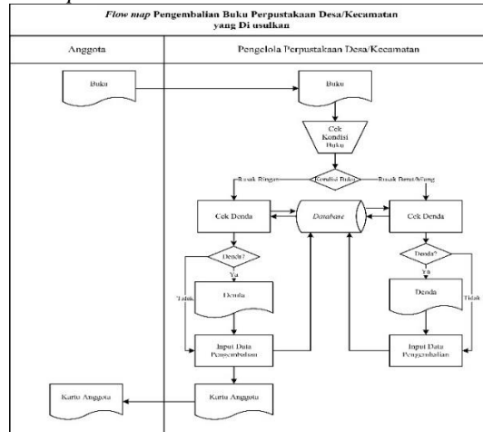
Gambar 6 Flow Map Pengembalian Buku Perpustakaan Desa/Kecamatan
