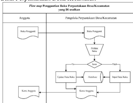
Gambar 7 Flow Map Penggantian Buku Perpustakaan Desa/Kecamatan
