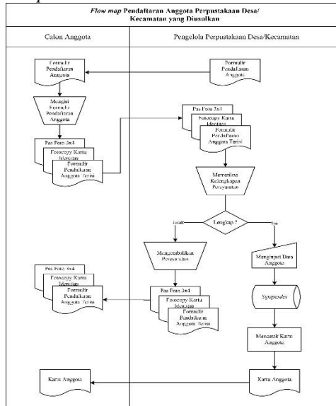
Gambar 3 Flow Map Pendaftaran Anggota Perpustakaan Desa/Kecamatan
