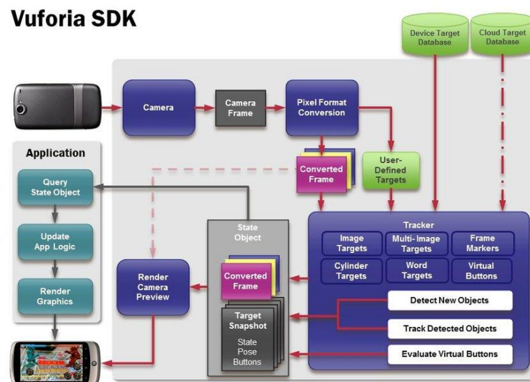
Gambar 2.6 Diagram Aliran Data Vuforia
