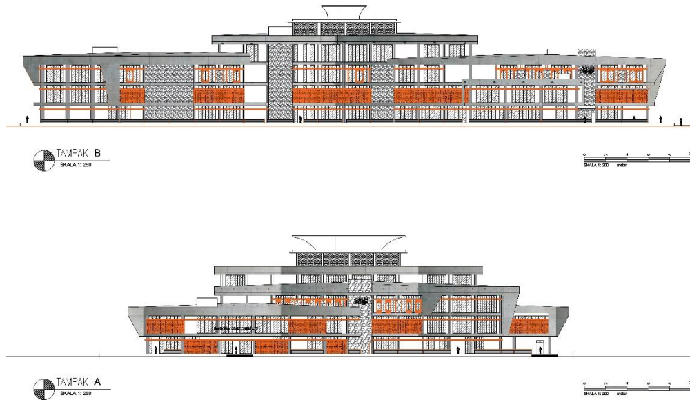
Gambar 1. 6.2.7 "Fasade Bangunan"
