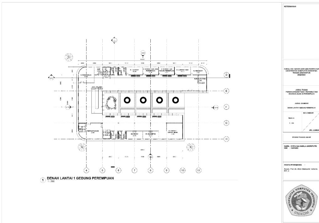
Gambar 6.9 Lt.1 Gedung Rehabilitasi Khusus Perempuan Sumber: Dokumentasi Pribadi
