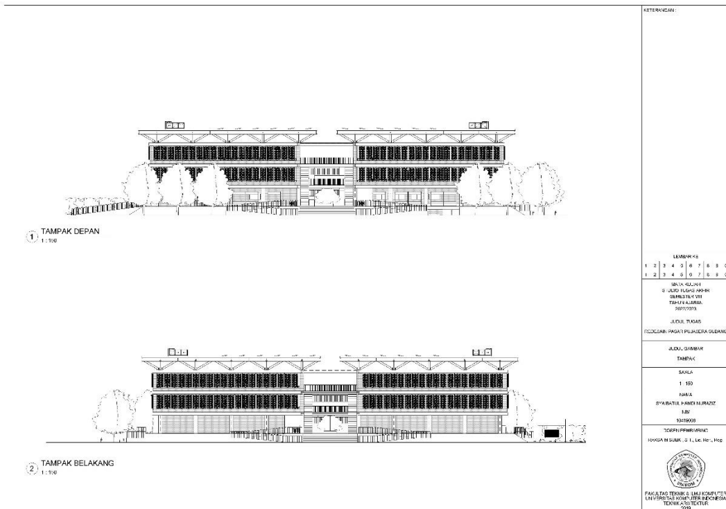
Tampak Depan
