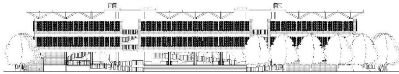
1 TAMPAK SAMPING KANAN 1:150
