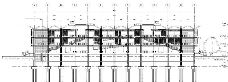
1 POTONGAN A-A 1:150
