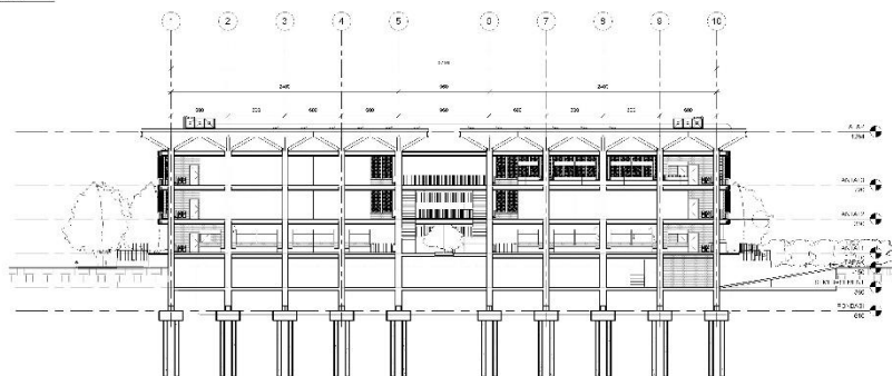
2 POTONGAN B-B 1:150
