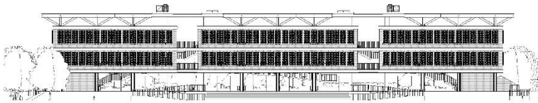
2 TAMPAK SAMPING KIRI 1:150
