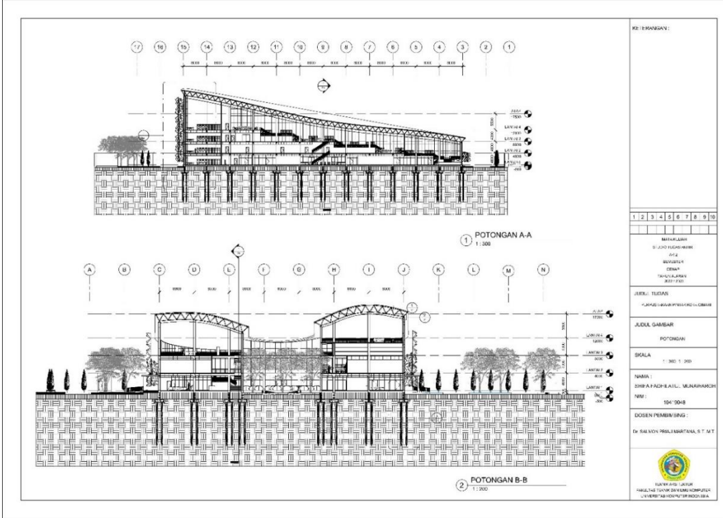
Gambar 6. 9 Potongan
