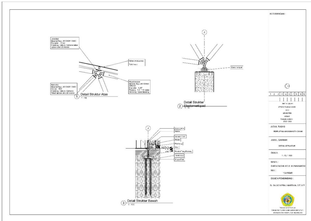
Gambar 6. 11 Detail Struktur
