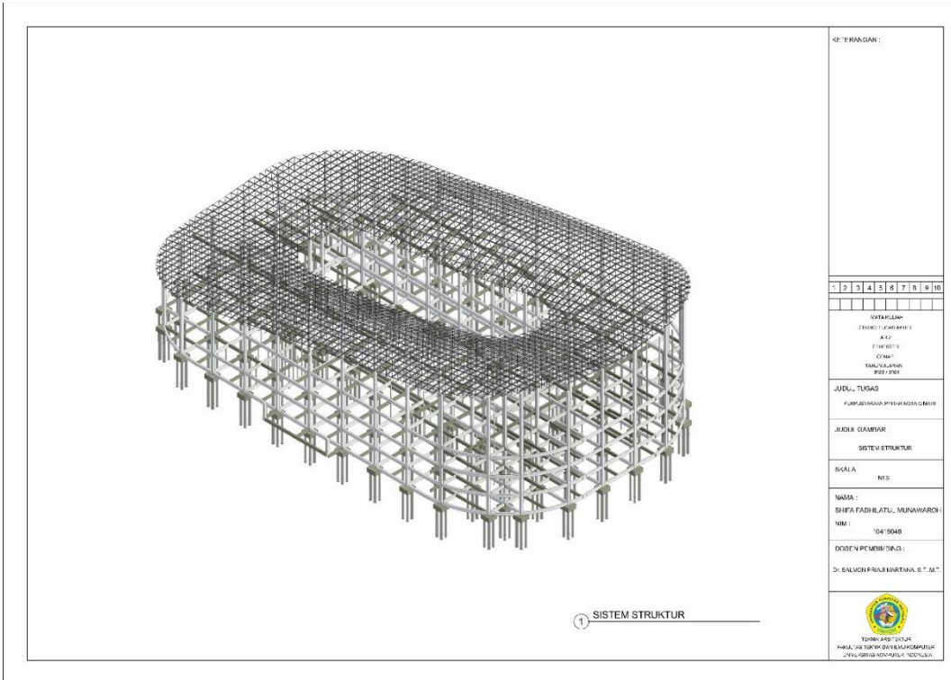
Gambar 6. 10 Sistem Struktur
