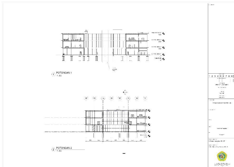
Gambar 6. 3 potongan 1 dan 2
