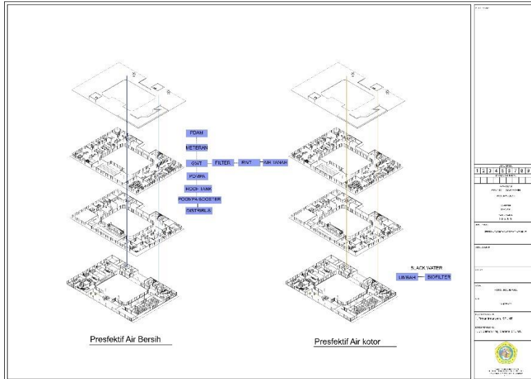
Gambar 6. 13 Utilitas
