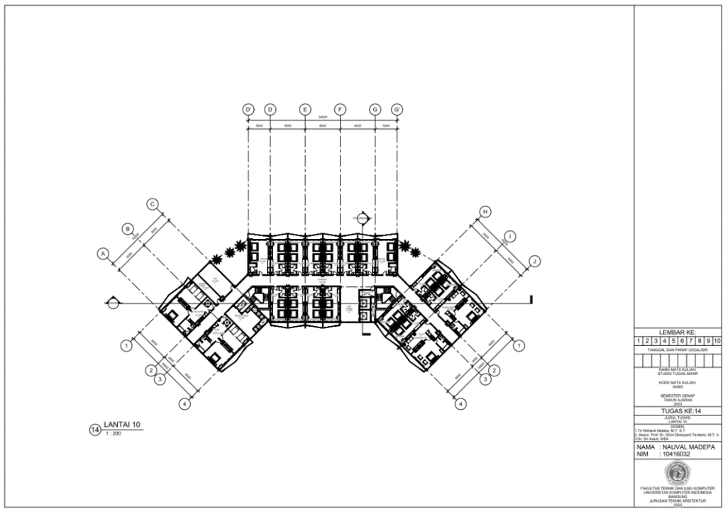
Gambar 6. 13 Lantai 10 (Sumber: Dokumentasi Pribadi, 2023)
