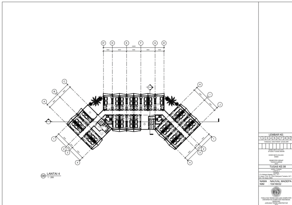
Gambar 6. 7 Lantai 4 (Sumber: Dokumentasi Pribadi, 2023)
