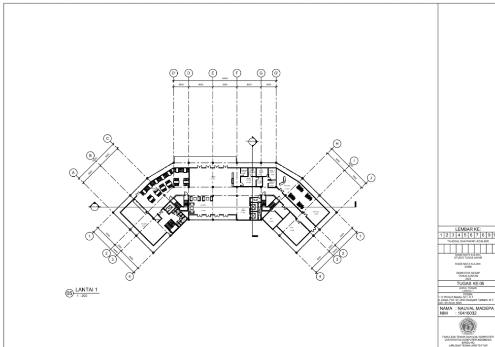
Gambar 6. 4 Lantai 1 (Sumber: Dokumentasi Pribadi, 2023)
