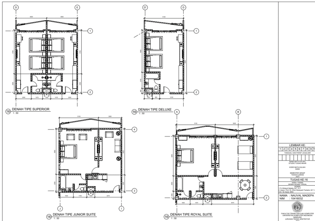
Gambar 6. 15 Denah Ruang Tipikal (Sumber: Dokumentasi Pribadi, 2023)
