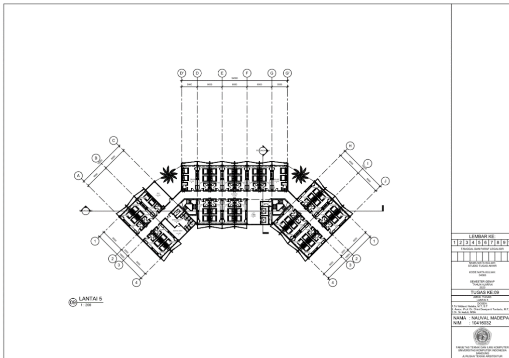
Gambar 6. 8 Lantai 5 (Sumber: Dokumentasi Pribadi, 2023)
