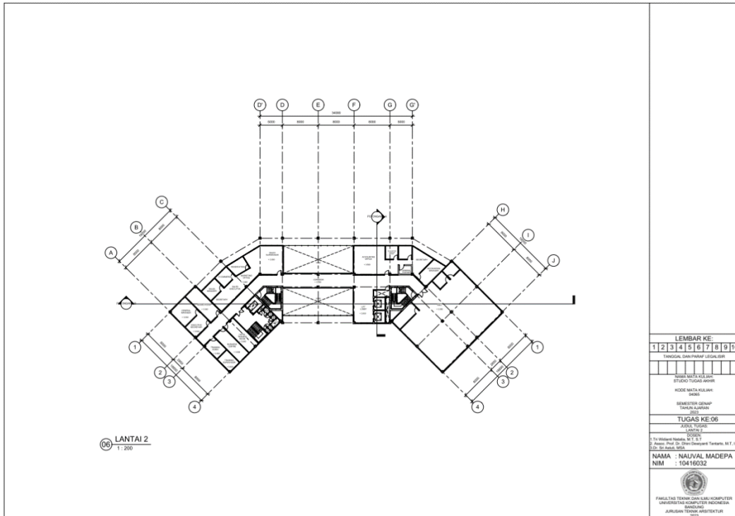
Gambar 6. 5 Lantai 2 (Sumber: Dokumentasi Pribadi, 2023)
