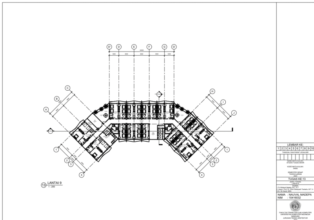
Gambar 6. 12 Lantai 9 (Sumber: Dokumentasi Pribadi, 2023)
