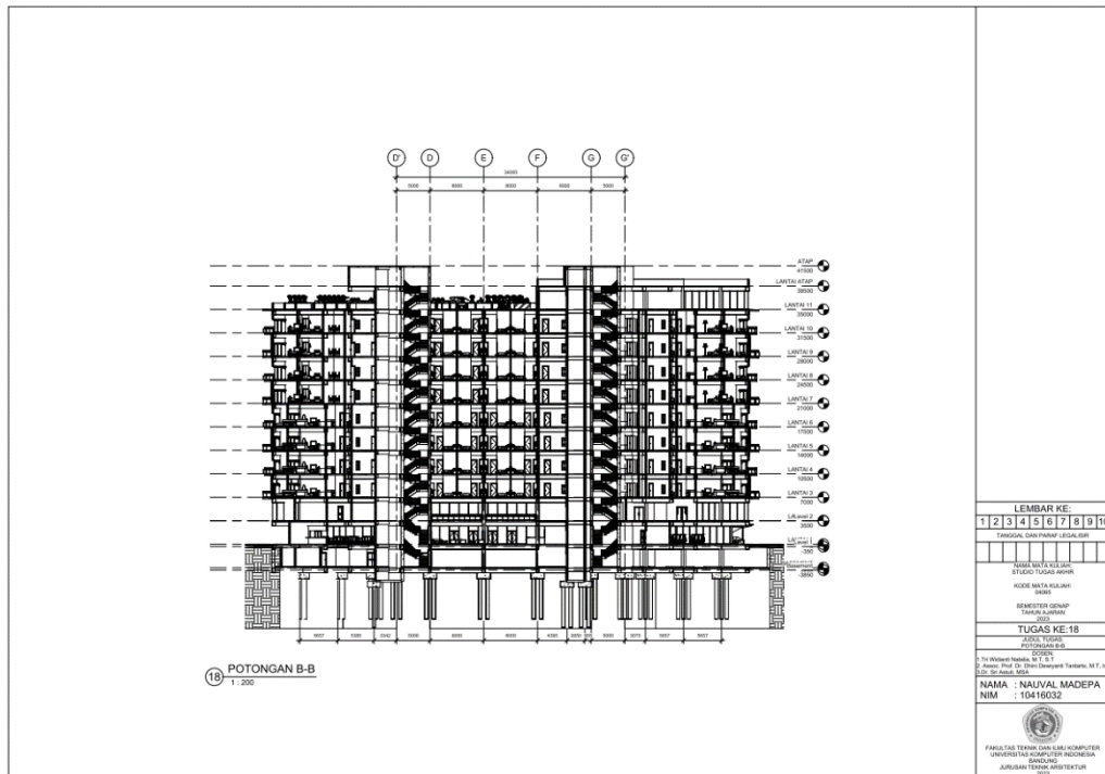
Gambar 6. 17 Potongan B-B (Sumber: Dokumentasi Pribadi, 2023)
