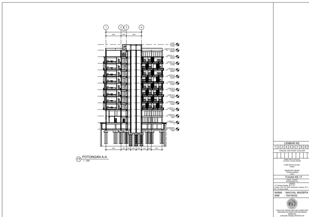
Gambar 6. 16 Potongan A-A (Sumber: Dokumentasi Pribadi, 2023)
