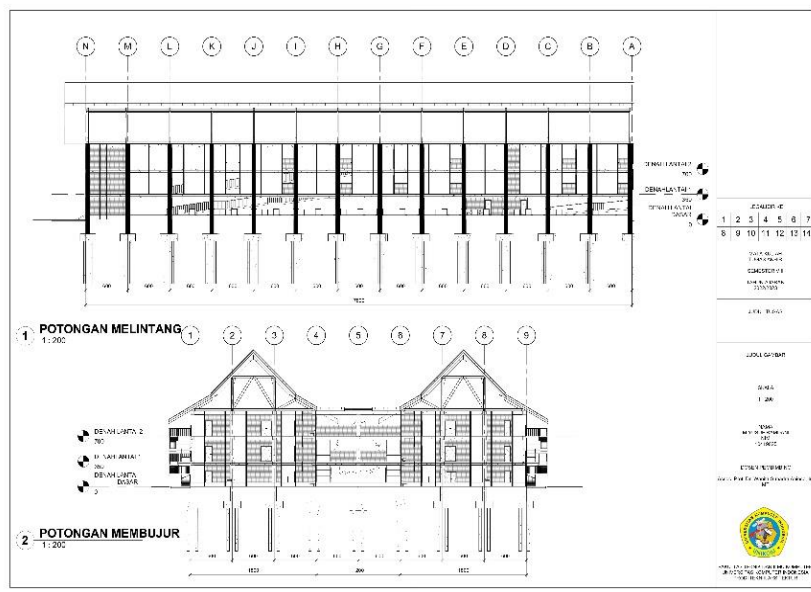
Gambar 6.8 Potongan
