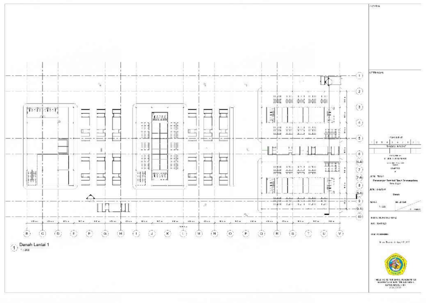
Gambar 6. 3 Denah lantai 1 Sumber : Dokumen Pribadi, 2023
