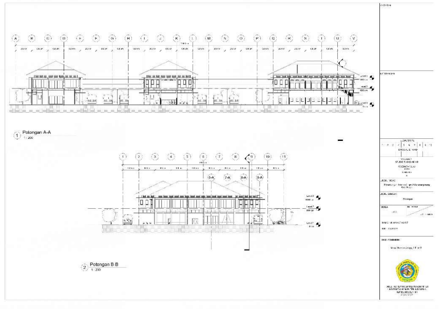
Gambar 6. 6 Tampak dan Potongan Masjid Sumber : Dokumen Pribadi, 2023
