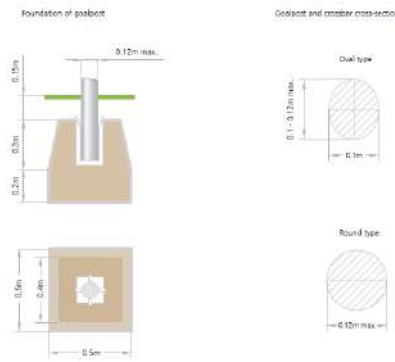
Gambar 2.4 Peletakan Pondasi Tiang gawang Pada Area Lapangan
