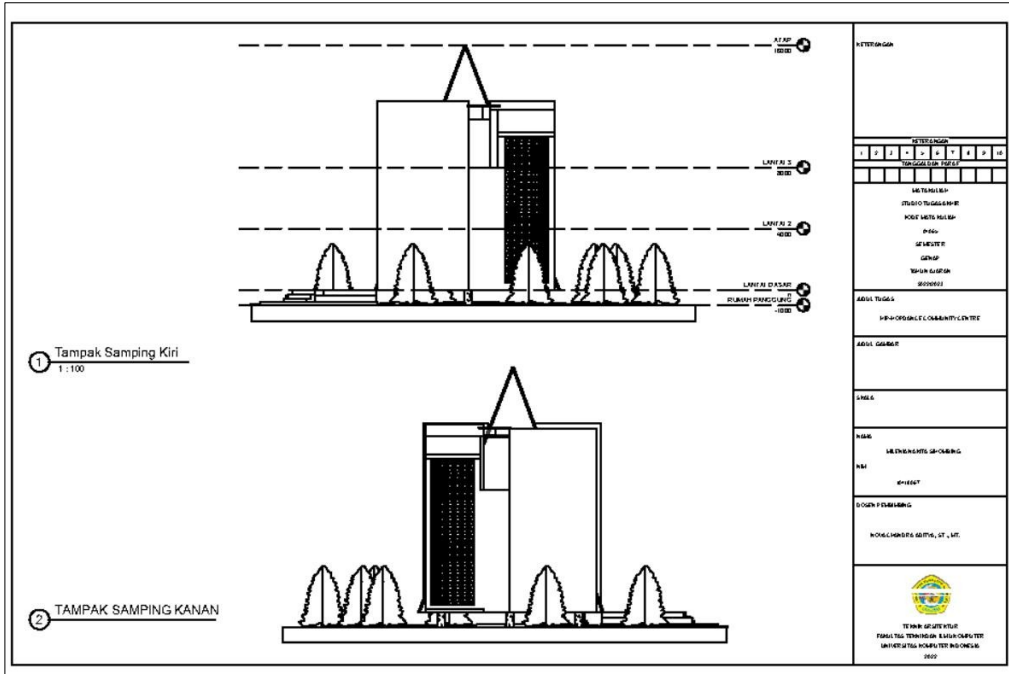
Gambar 6. 4 Tampak Samping Kanan dan Kiri Sumber : Dokumen Pribadi, 2023
