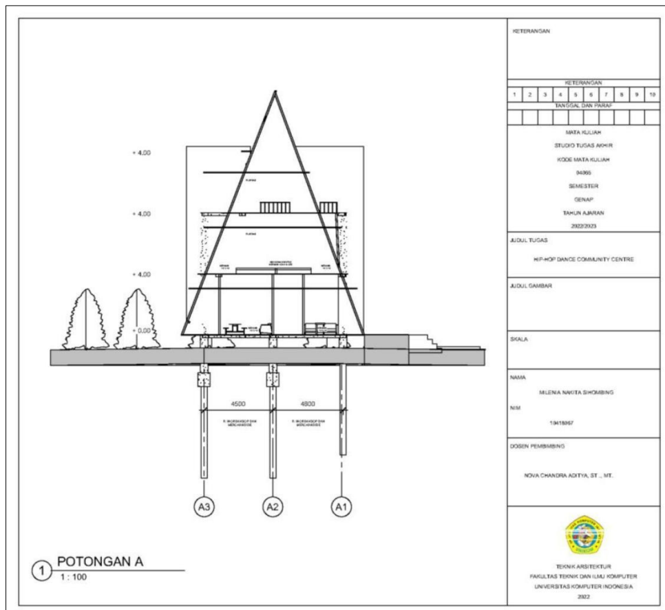
Gambar 6. 5 Potongan A Sumber : Dokumen Pribadi, 2023
