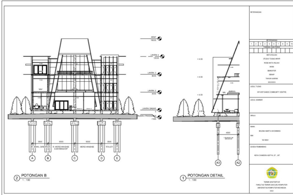
Gambar 6. 6 Potongan B dan Potongan detail
