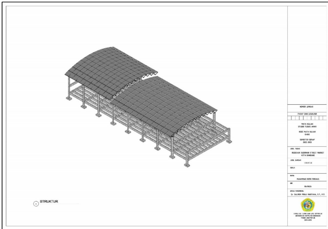
Gambar 6. 9 Struktur Sumber : Dokumen Pribadi
