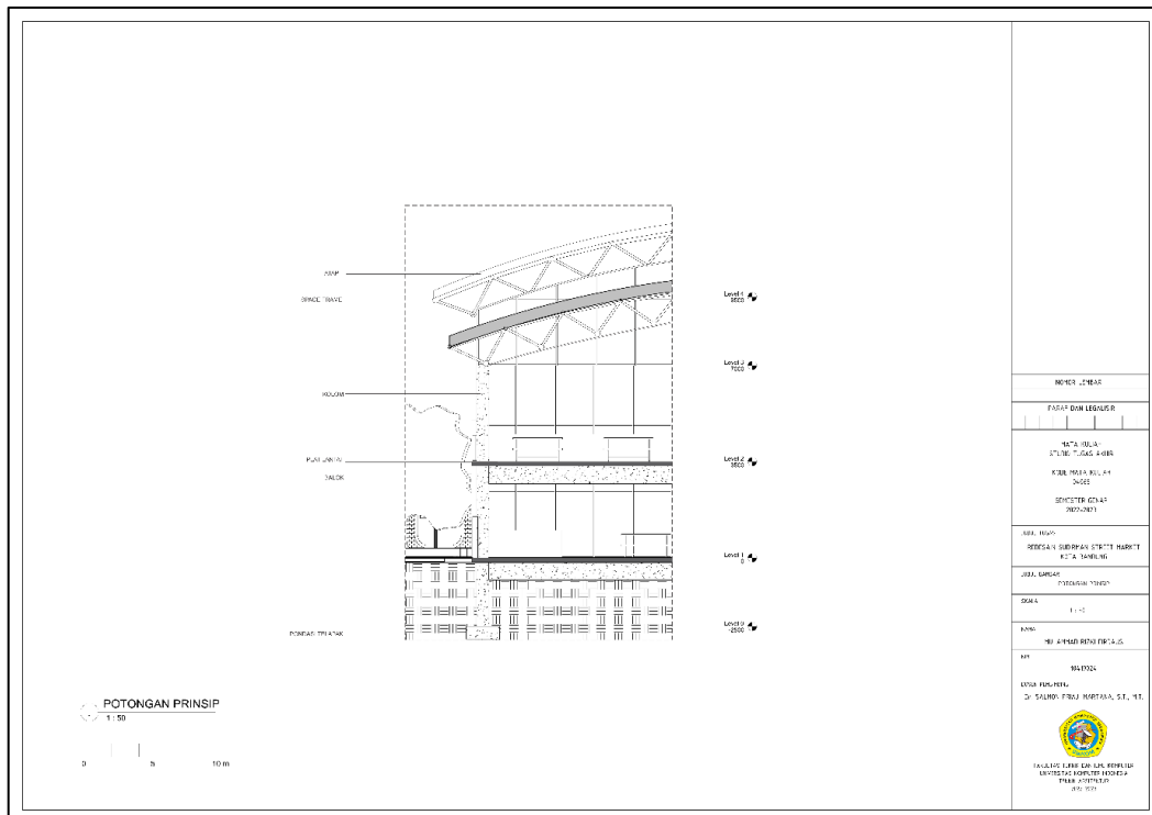
Gambar 6. 8 Potongan Prinsip Sumber : Dokumen Pribadi
