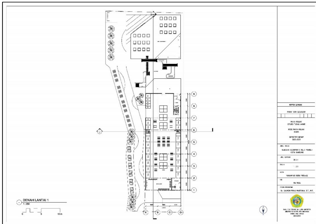
Gambar 6. 3 Denah Lantai 1 Sumber : Dokumen Pribadi
