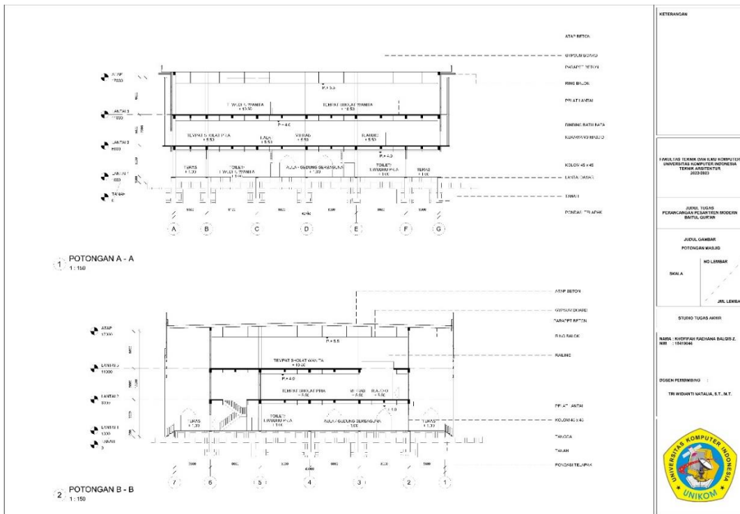
Gambar 6. 6 Potongan Masjid (Sumber : Dokumen Pribadi)
