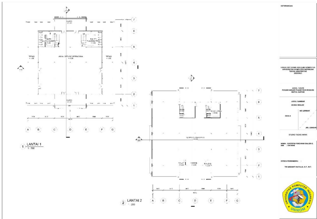
Gambar 6. 3 Denah Masjid Lantai 1 dan 2 (Sumber : Dokumen Pribadi)
