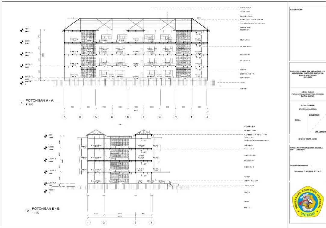
Gambar 6. 16 Potongan Asrama (Sumber : Dokumen Pribadi)
