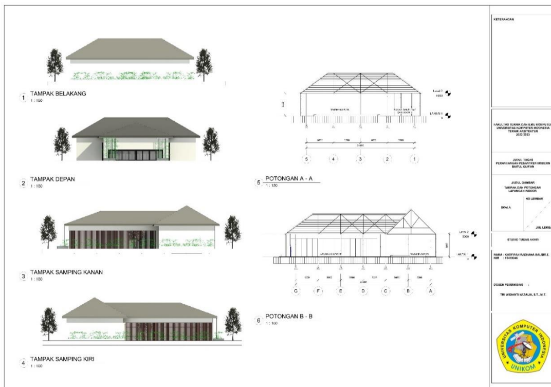
Gambar 6. 45 Tampak dan Potongan Sarana Olahraga Indoor
