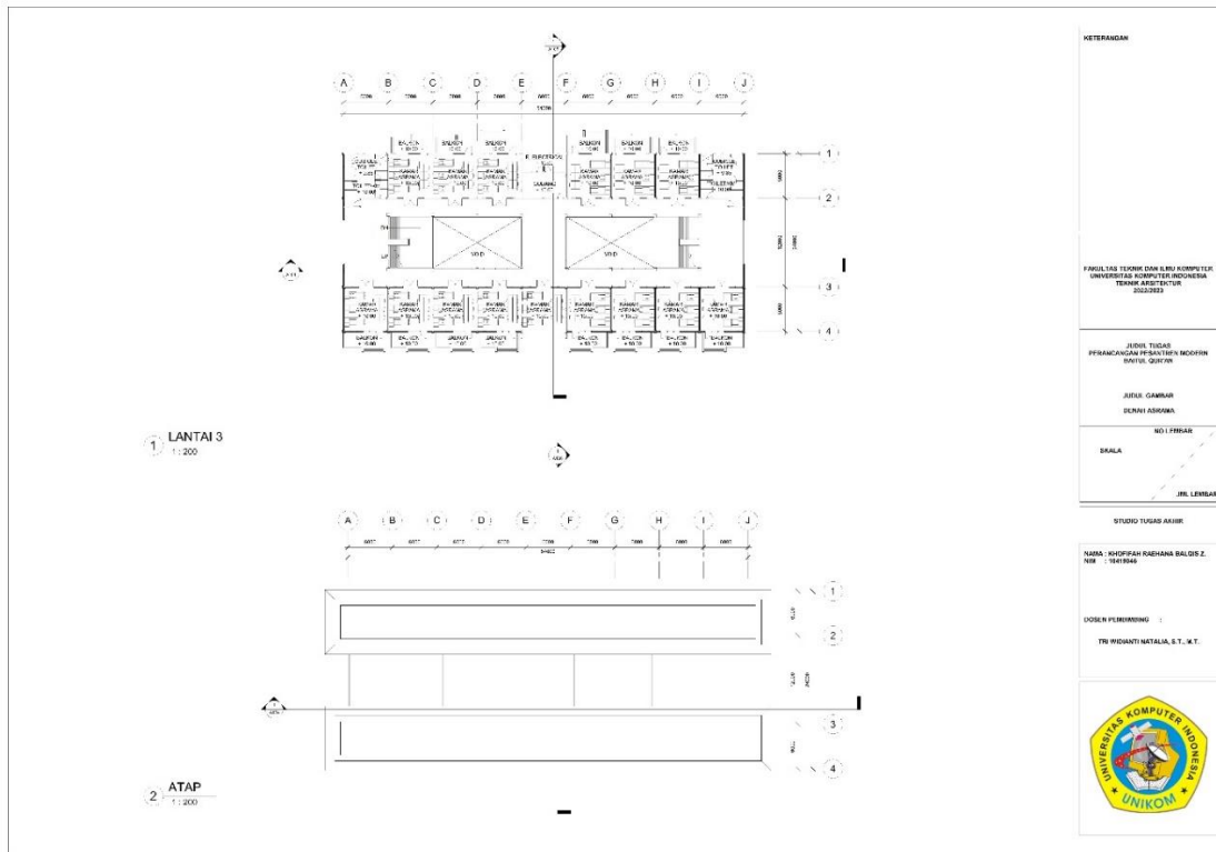
Gambar 6. 14 Denah Asrama Lantai 3 dan Atap (Sumber : Dokumen Pribadi)
