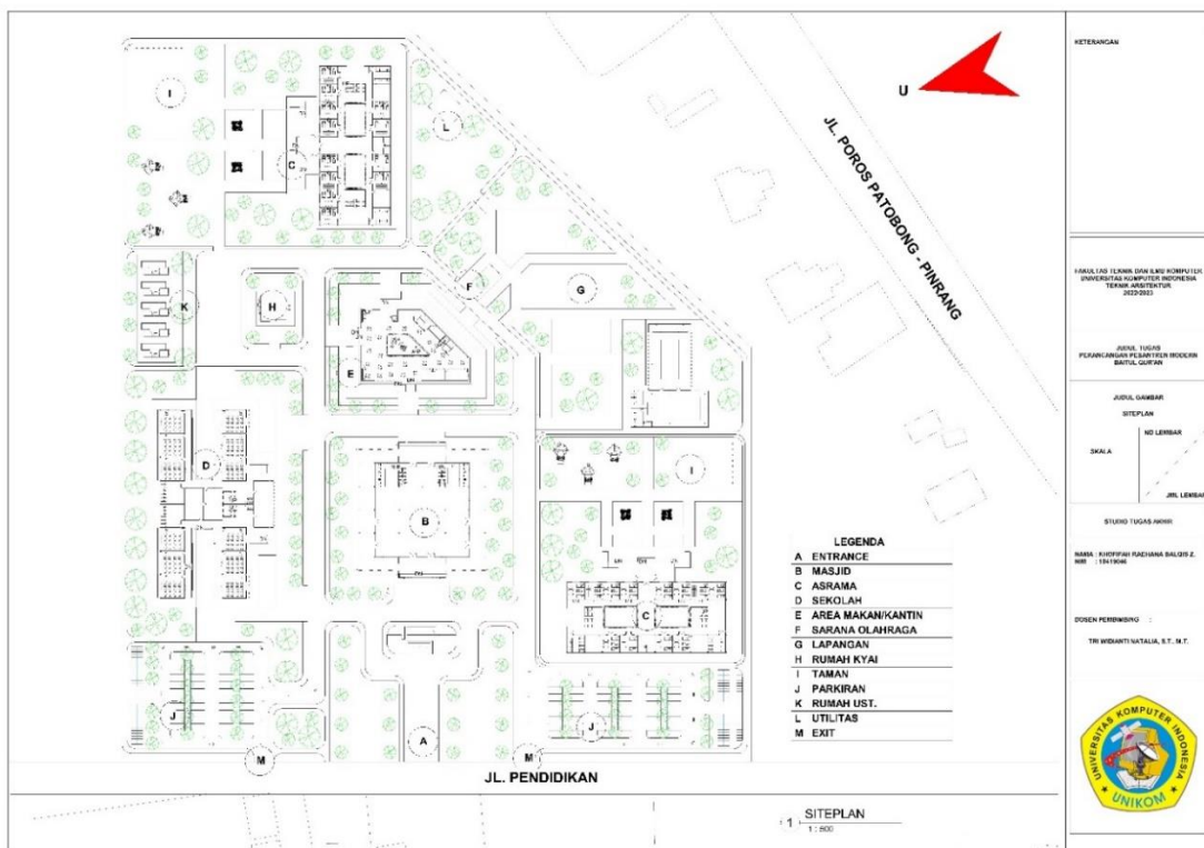
Gambar 6. 2 Siteplan (Sumber : Dokumen Pribadi)
