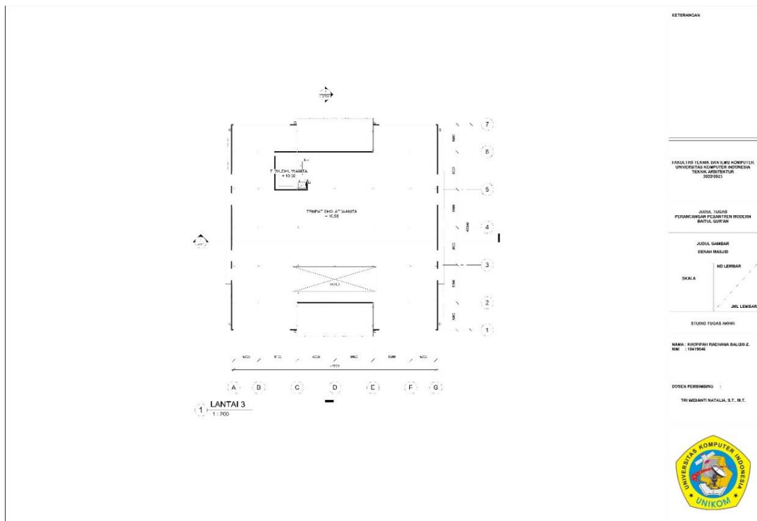
Gambar 6. 4 Denah Masjid Lantai 3 (Sumber : Dokumen Pribadi)
