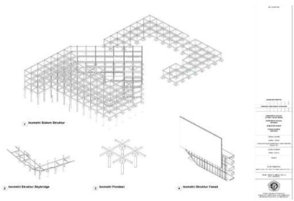
Gambar 6. 9 Sistem Struktur
