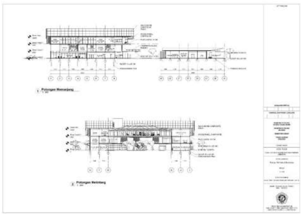
Gambar 6. 7 Potongan
