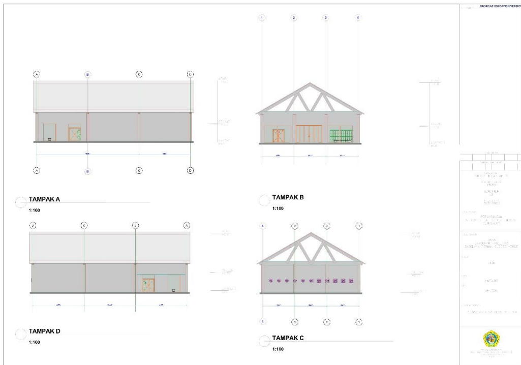
Gambar 6.24 Tampak
