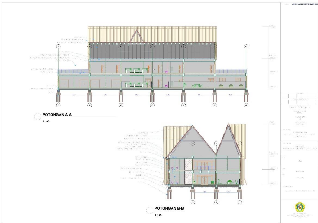
Gambar 6.10 Potongan
