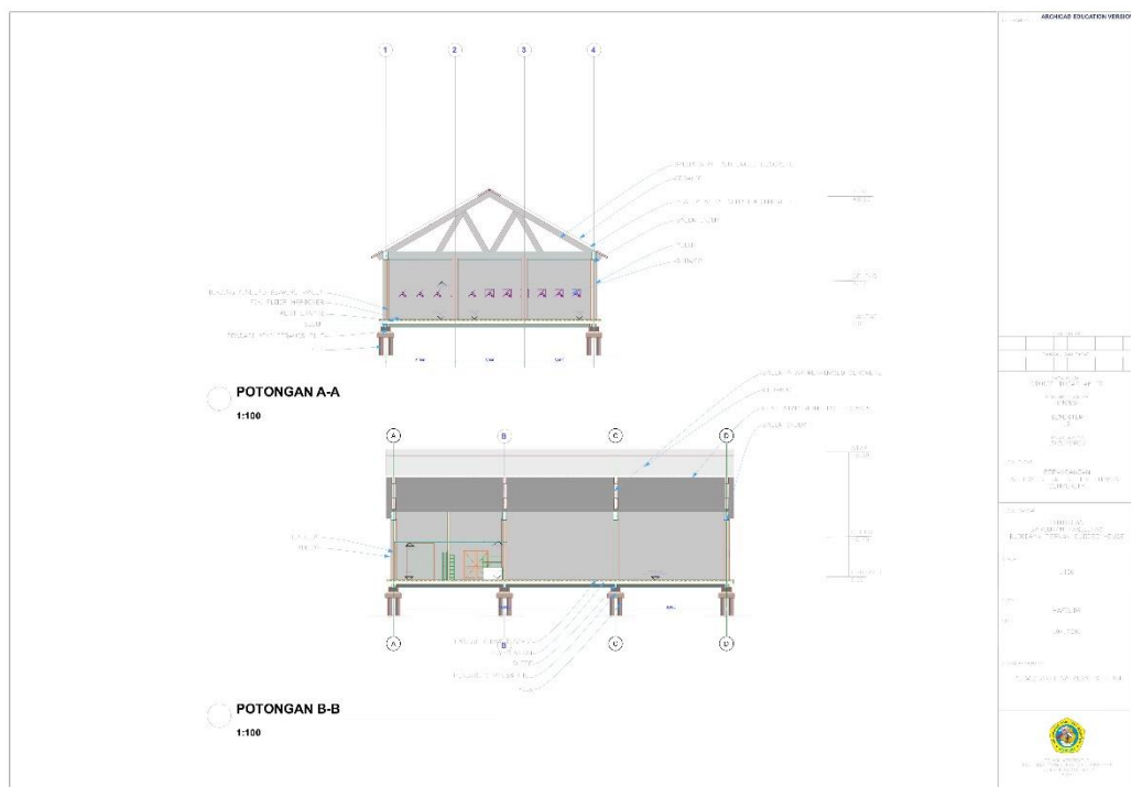
Gambar 6.23 Potongan
