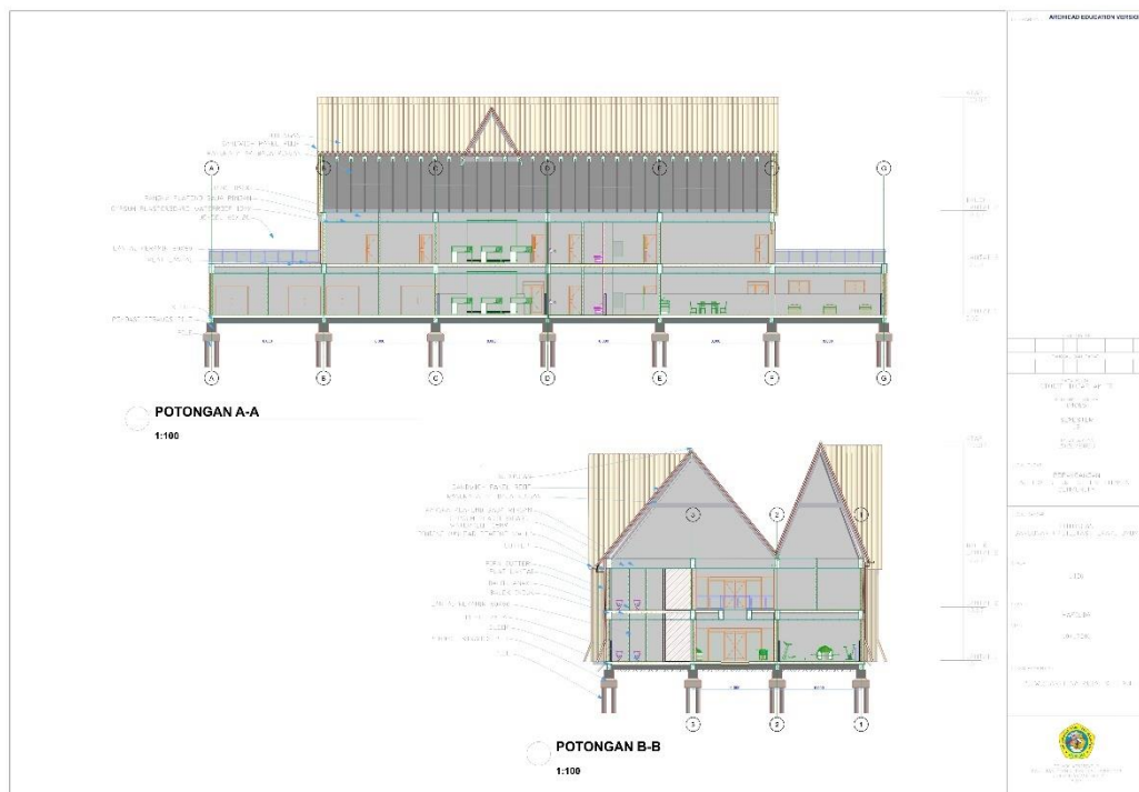
Gambar 6.7 Potongan Fasilitas Terapi Umum
