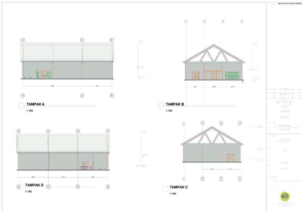
Gambar 6.21 Tampak
