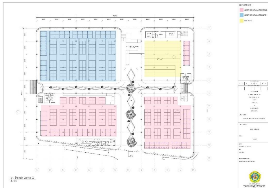
Gambar 6.4 Denah lantai 1 Sumber gambar : Dokumentasi Pribadi
