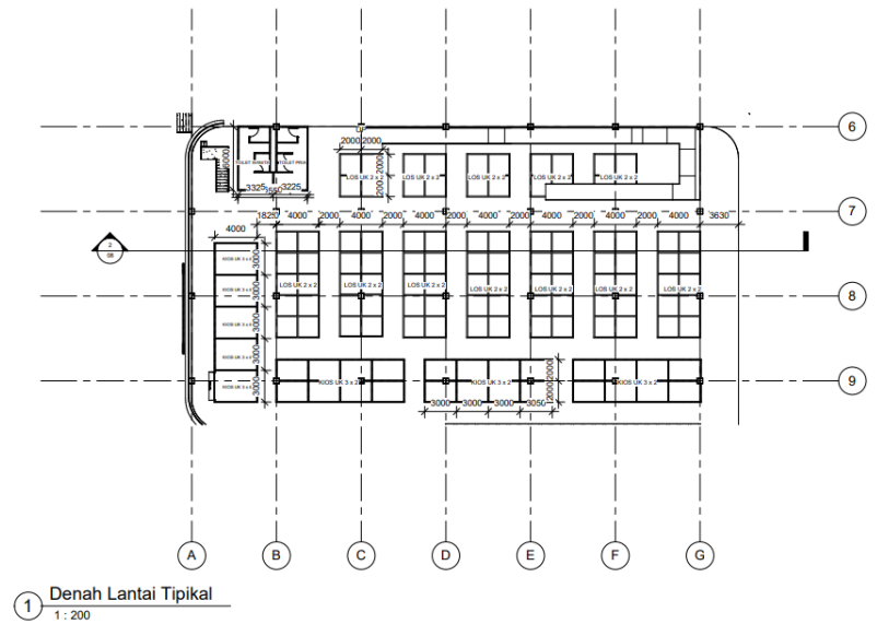
Gambar 6.9 Denah area Kios Sumber gambar : Dokumentasi Pribadi
