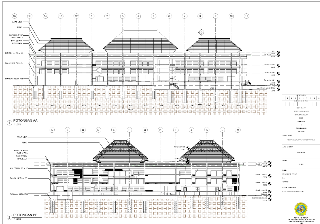
Gambar 6.8 Potongan Bangunan Sumber gambar : Dokumentasi Pribadi
