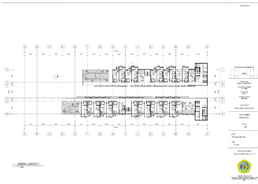
Gambar 6.9 Denah Lantai 7 (Dokumentasi Pribadi, 2023)
