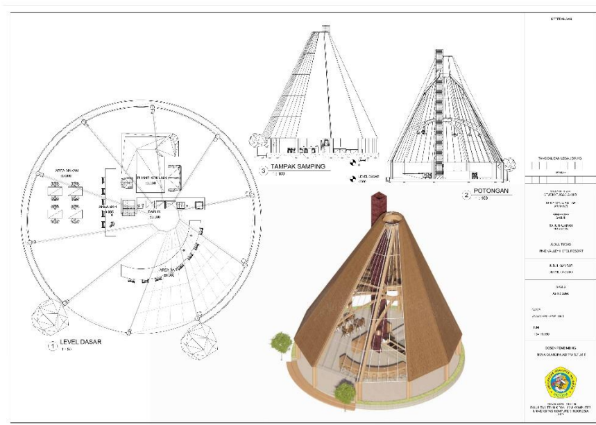
Gambar 6.21 Detail Gazebo (Dokumentasi Pribadi, 2023)
