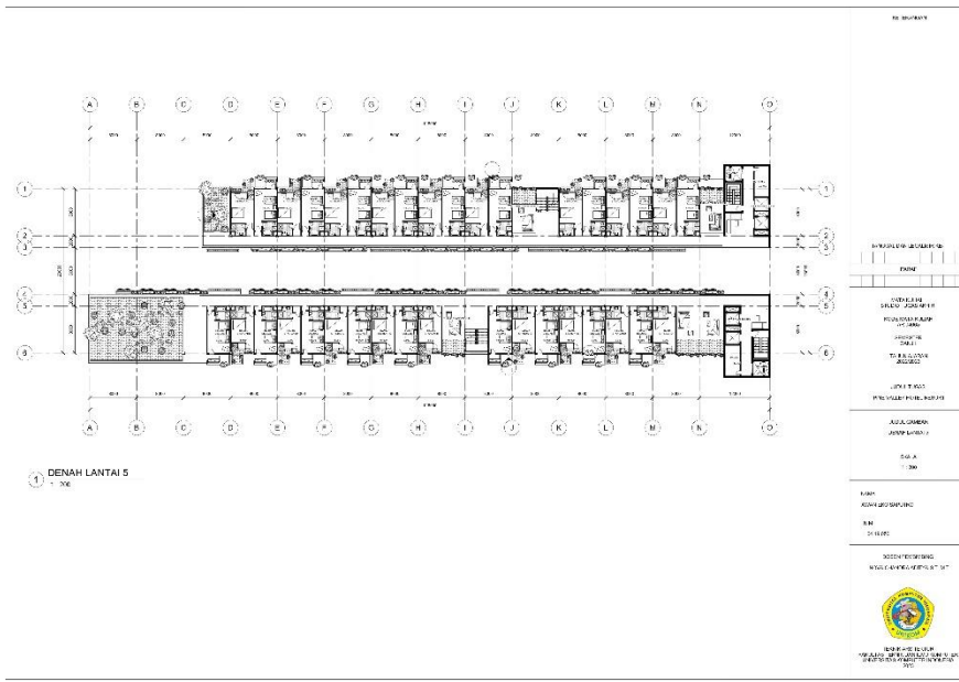
Gambar 6.7 Denah Lantai 5 (Dokumentasi Pribadi, 2023)
