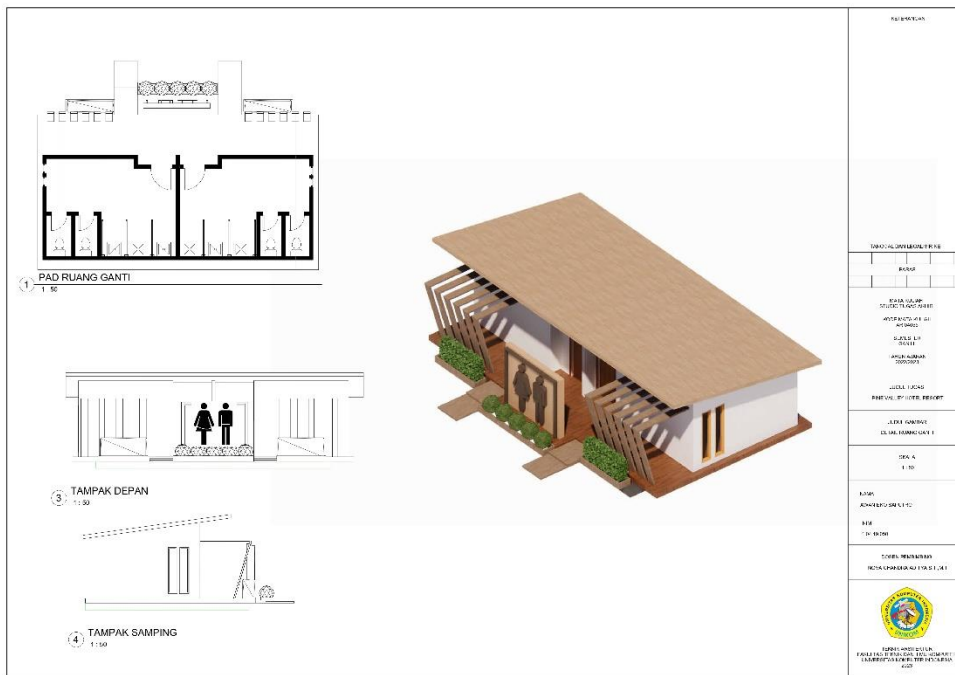
Gambar 6.23 Detail Ruang Ganti (Dokumentasi Pribadi, 2023)
