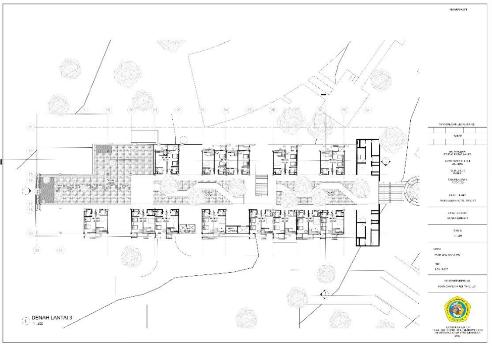
Gambar 6.5 Denah Lantai 3 (Dokumentasi Pribadi, 2023)
