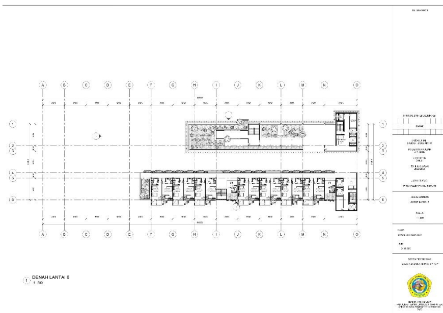
Gambar 6.10 Denah Lantai 8 (Dokumentasi Pribadi, 2023)
