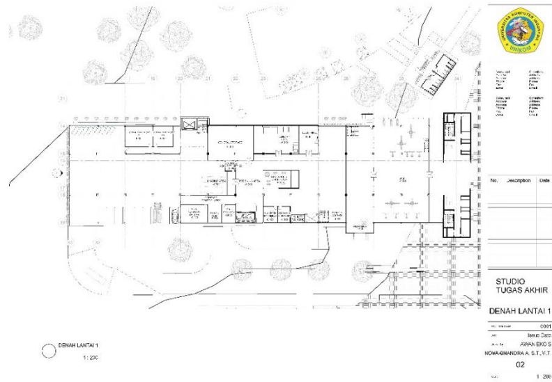
Gambar 6.3 Denah lantai 1 (Dokumentasi Pribadi, 2023)
