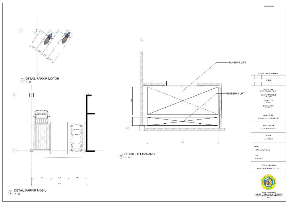
Gambar 6.18 Detail Arsitektur 2 (Dokumentasi Pribadi, 2023)
