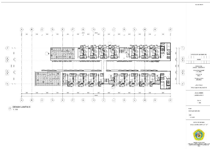
Gambar 6.8 Denah Lantai 6 (Dokumentasi Pribadi, 2023)
