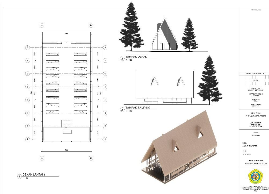
Gambar 6.25 Detail Multi Functional Hall (Dokumentasi Pribadi, 2023)
