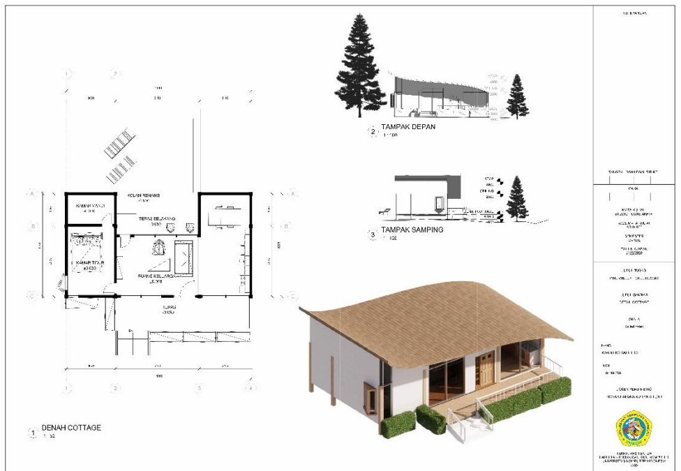
Gambar 6.20 Detail Cottage (Dokumentasi Pribadi, 2023)
