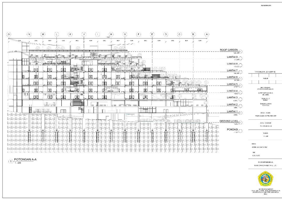
Gambar 6.15 Potongan A-A (Dokumentasi Pribadi, 2023)
