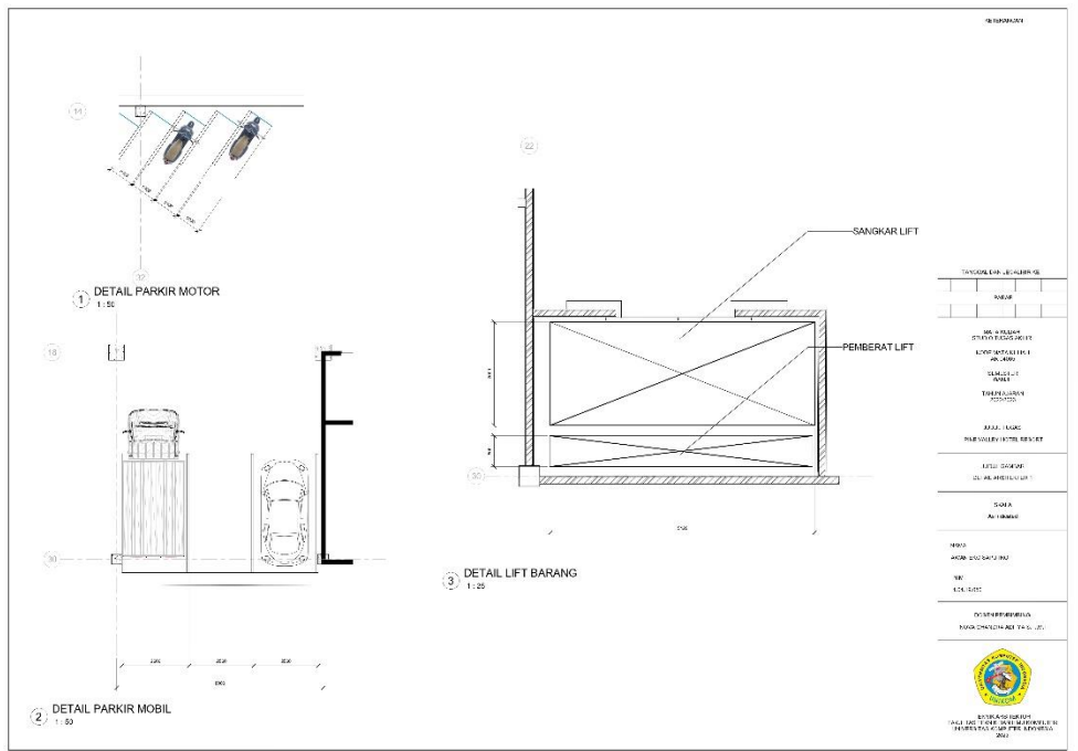
Gambar 6.19 Detail Arsitektur 2 (Dokumentasi Pribadi, 2023)
