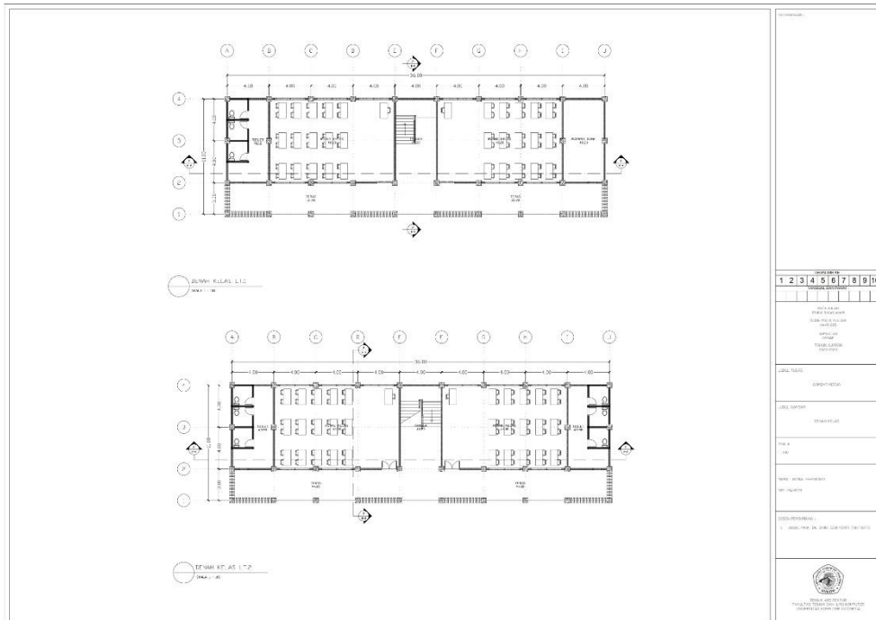
Gambar 6. 6 Denah Kelas
