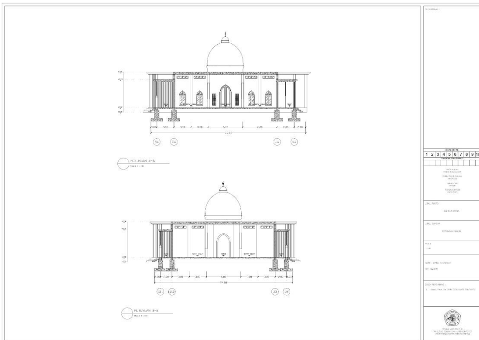
Gambar 6. 4 Potongan Masjid
