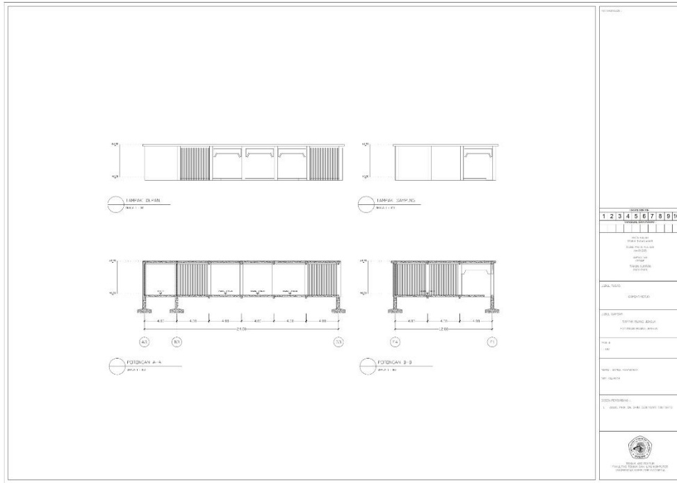
Gambar 6. 17 Tampak & Potongan Ruang Jenguk
