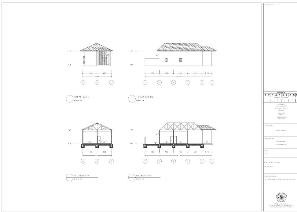
Gambar 6. 23 Tampak & Potongan
