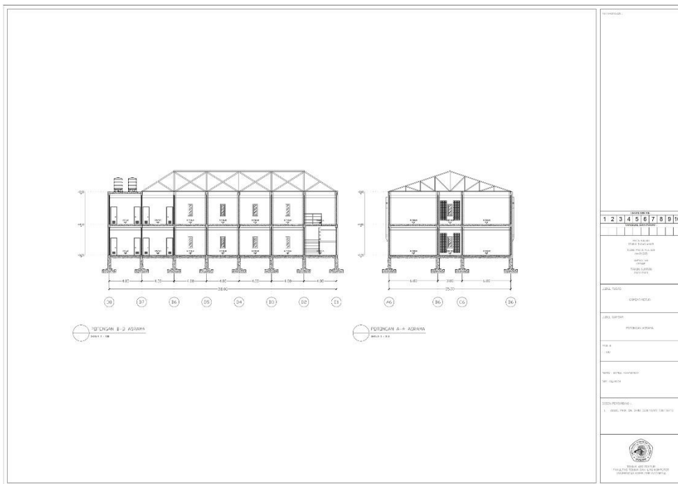
Gambar 6. 10 Potongan Asrama
