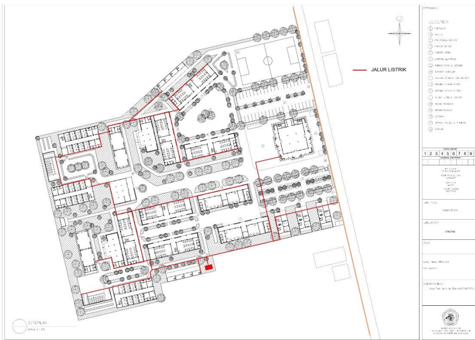
Gambar 6. 24 Utilitas Kelistrikan
