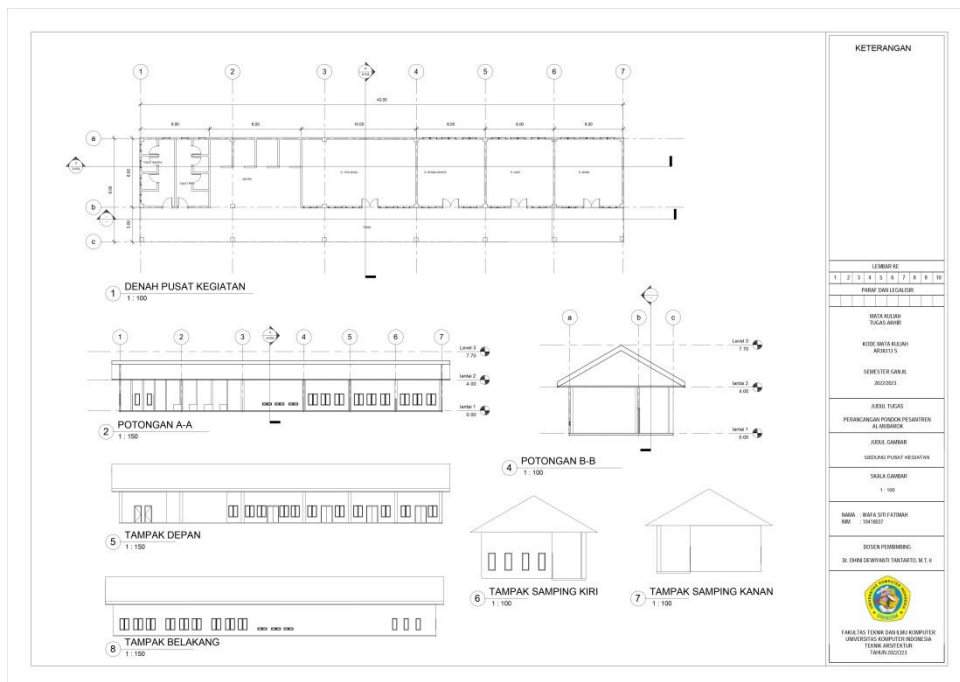
Gambar 6. 10 gedung pusat kegiatan sumber: Dokumen Pribadi
