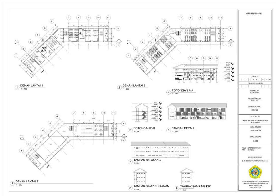
Gambar 6. 6 Sekolah MA sumber: Dokumen Pribadi
