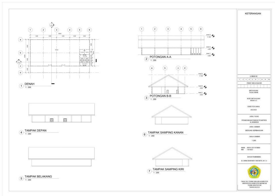
Gambar 6. 8 gedung serbaguna sumber: Dokumen Pribadi
