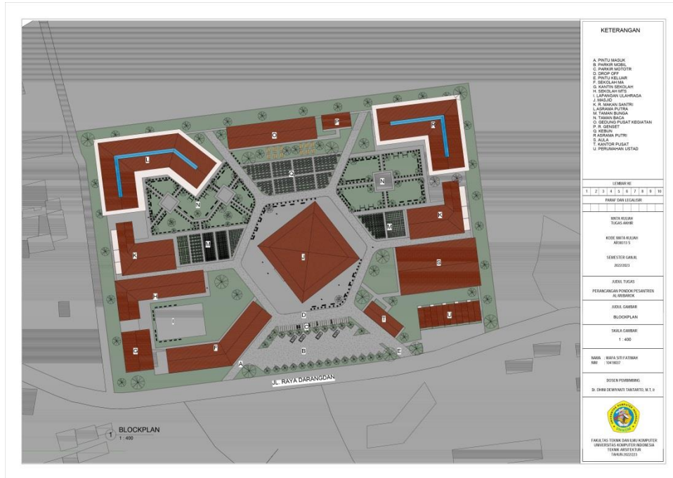
Gambar 6. 1 Blockplan sumber: Dokumen Pribadi
