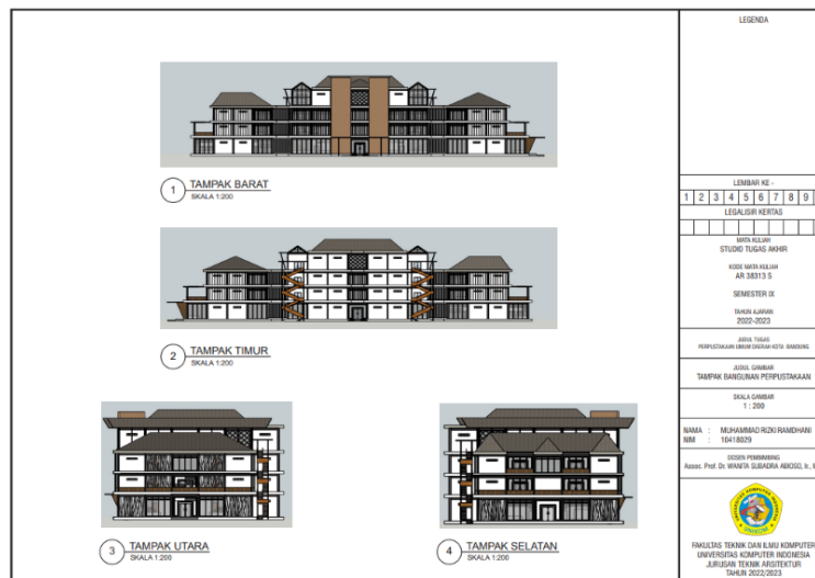
Gambar 6.4 Tampak Bangunan
