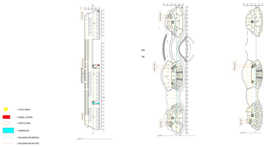
Gambar 6. 7 Utilitas Air bersih, air kotor, dan listrik sumber: penulis
