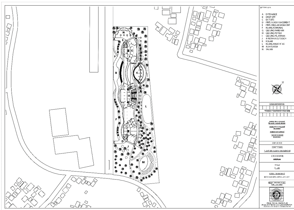
Gambar 6. 2 Siteplan Penulis
