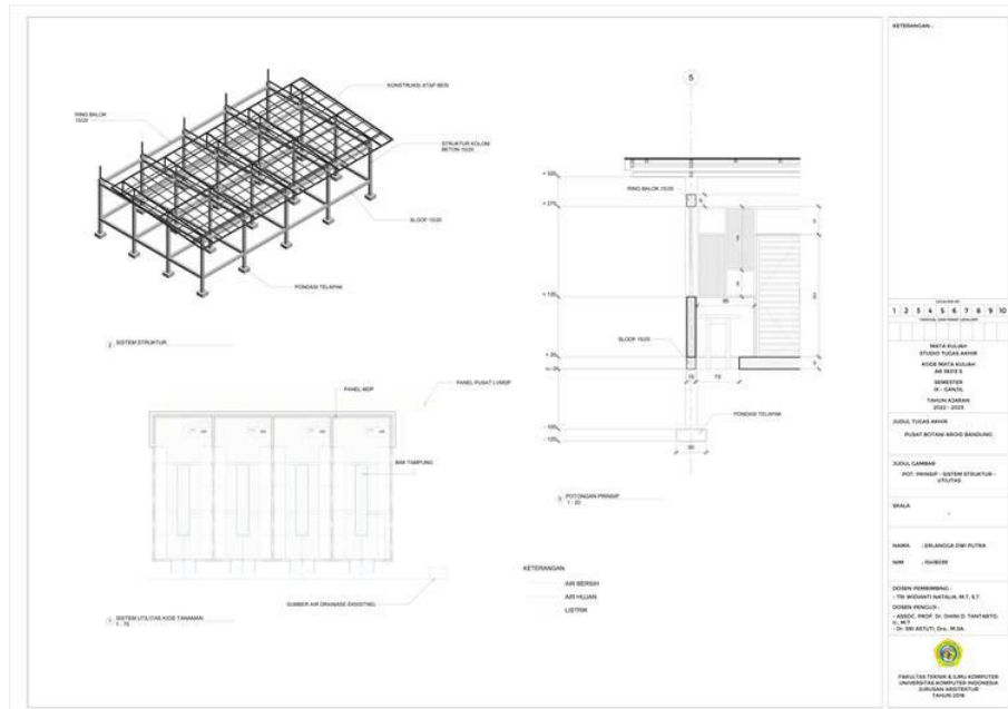
Gambar 6. 13 Pot. Prinsip, Sistem Struktur & Utilitas
