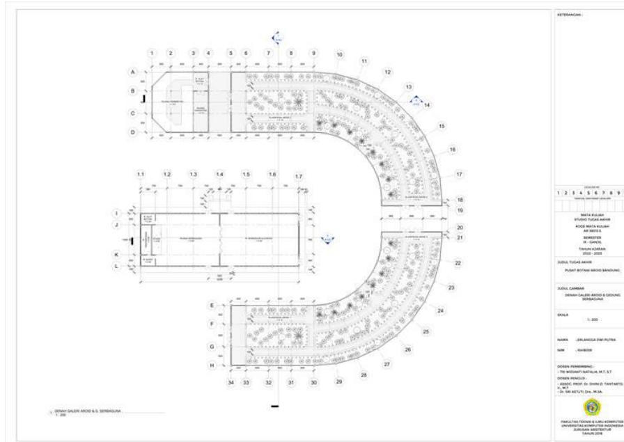
Gambar 6. 5 Denah Bangunan Zona Aroid
