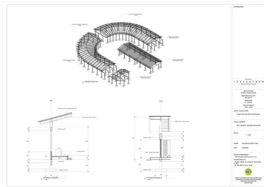
Gambar 6. 11 Pot. Prinsip & Sistem Struktur Zona Aroid
