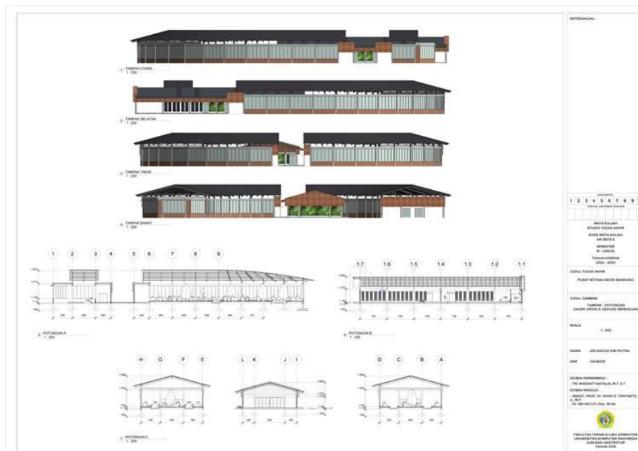
Gambar 6. 6 Tampak & Potongan Bangunan Zona Aroid
