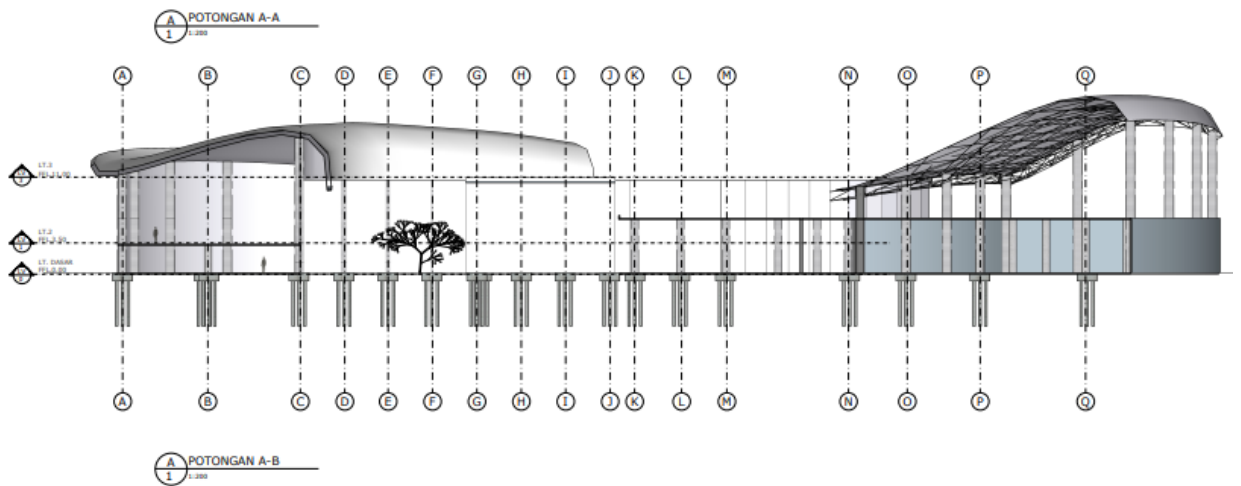
Gambar 6. 10 Potongan 2
