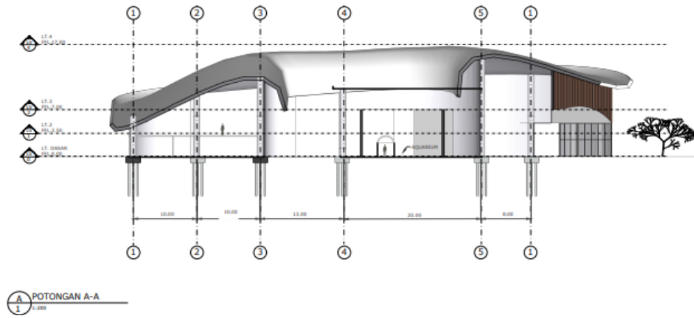
Gambar 6. 9 Potongan 1
