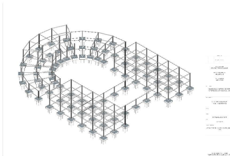
GAMBAR 49 Sistem Struktur
