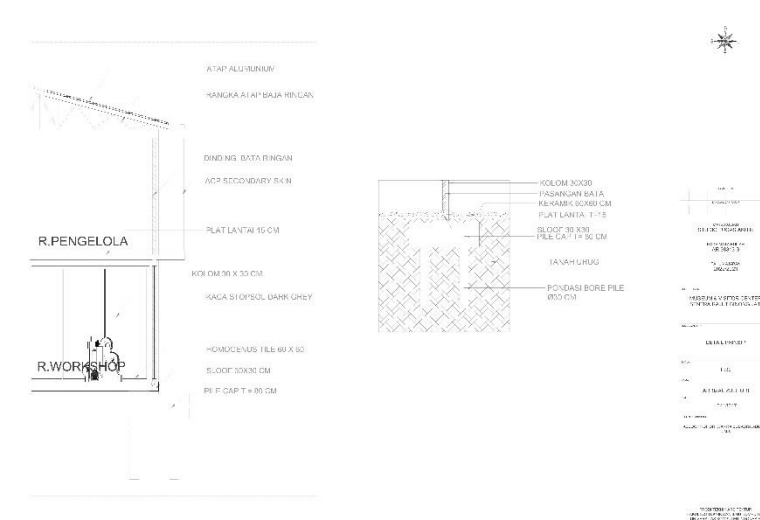
GAMBAR 48 potongan Prinsip
