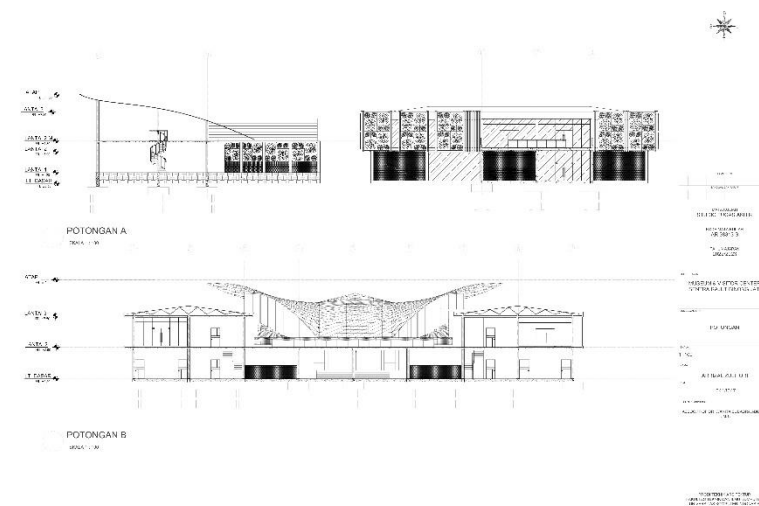
GAMBAR 47 Potongan
