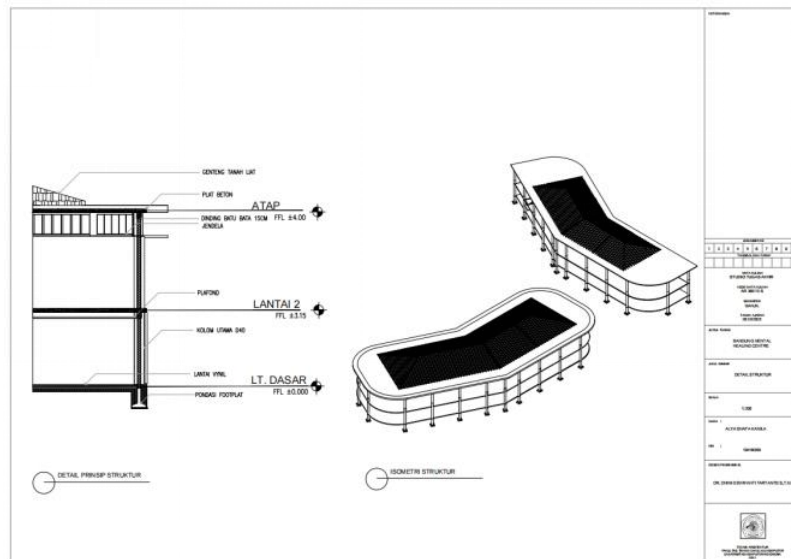
Gambar 6. 7 Detail Struktur
