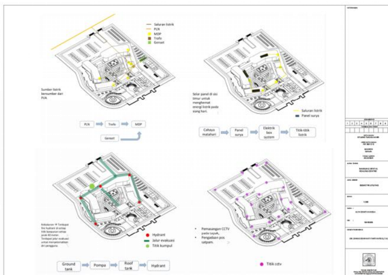
Gambar 6. 9 Utilitas
