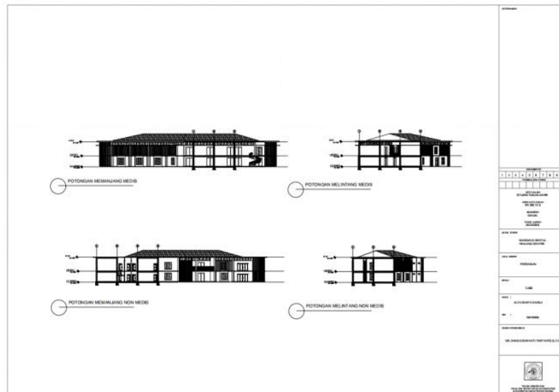
Gambar 6. 6 Potongan
