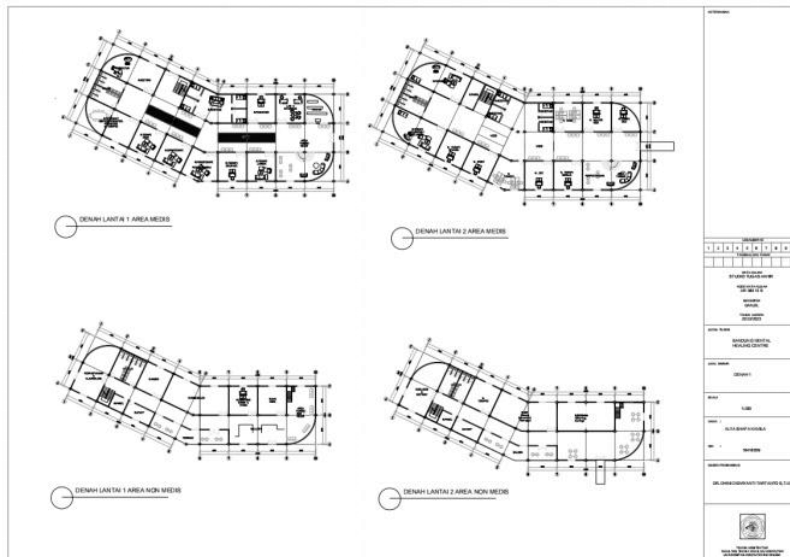
Gambar 6. 3 Denah Bangunan Medis dan Non-Medis
