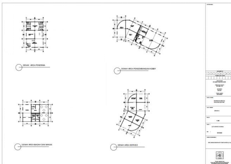
Gambar 6. 4 Denah Bangunan Penerima, Mushola, Hobby dan Servis
