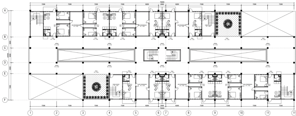
Gambar 6. 6 Denah Lantai 4 Sumber: Hasil Rancangan Penulis, 2022
