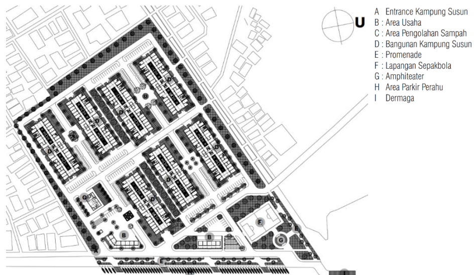
Gambar 6. 2 Site Plan Sumber: Hasil Rancangan Penulis, 2022
