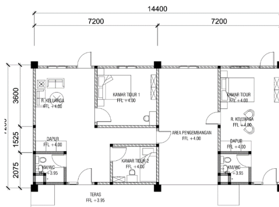
Gambar 6. 8 Denah Parsial Hunian Sumber: Hasil Rancangan Penulis, 2022
