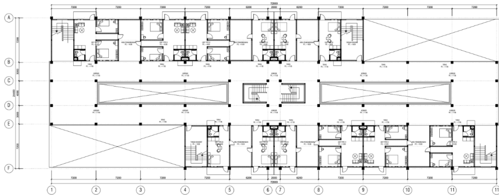
Gambar 6. 7 Denah Lantai 5 Sumber: Hasil Rancangan Penulis, 2022
