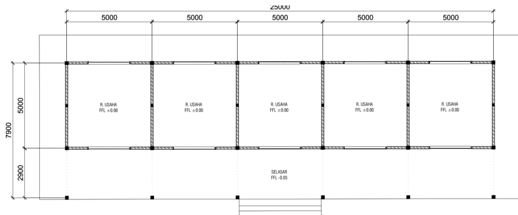
Gambar 6. 11 Denah Ruang Usaha Sumber: Hasil Rancangan Penulis, 2022
