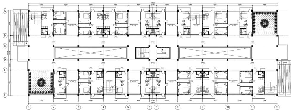
Gambar 6. 4 Denah Lantai 2 Sumber: Hasil Rancangan Penulis, 2022
