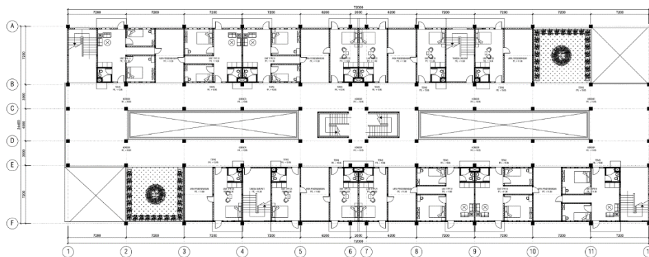
Gambar 6. 5 Denah Lantai 3 Sumber: Hasil Rancangan Penulis, 2022
