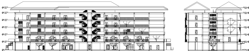
Gambar 6. 10 Potongan Sumber: Hasil Rancangan Penulis, 2022
