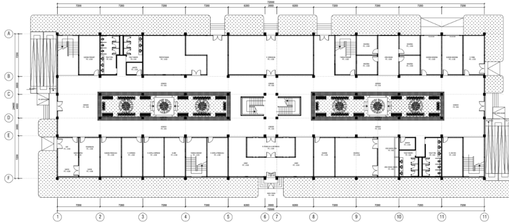
Gambar 6. 3 Denah Lantai Dasar Sumber: Hasil Rancangan Penulis, 2022
