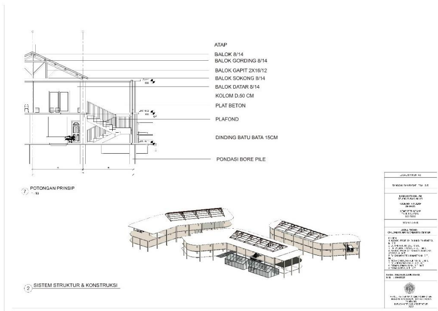
Gambar 6. 6 Sistem Struktur dan Konstruksi Sumber: Dokumen Pribadi
