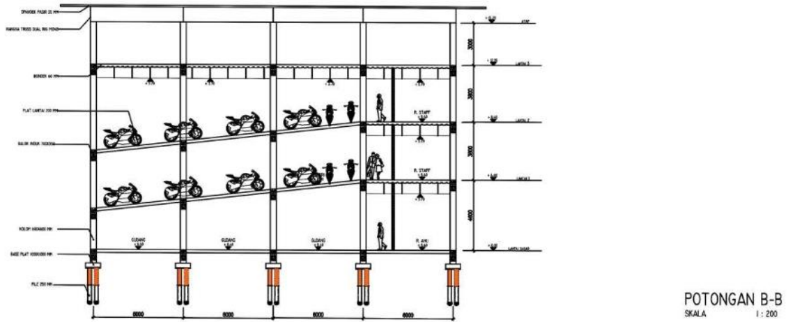
Gambar 6. 11 Potongan B-B
