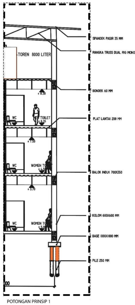
Gambar 6. 22 Potongan Prinsip 1
