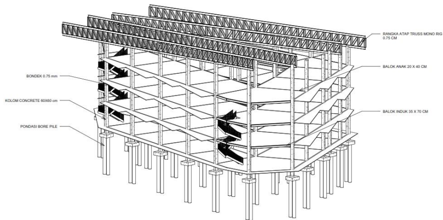
Gambar 6. 21 Sistem Struktur
