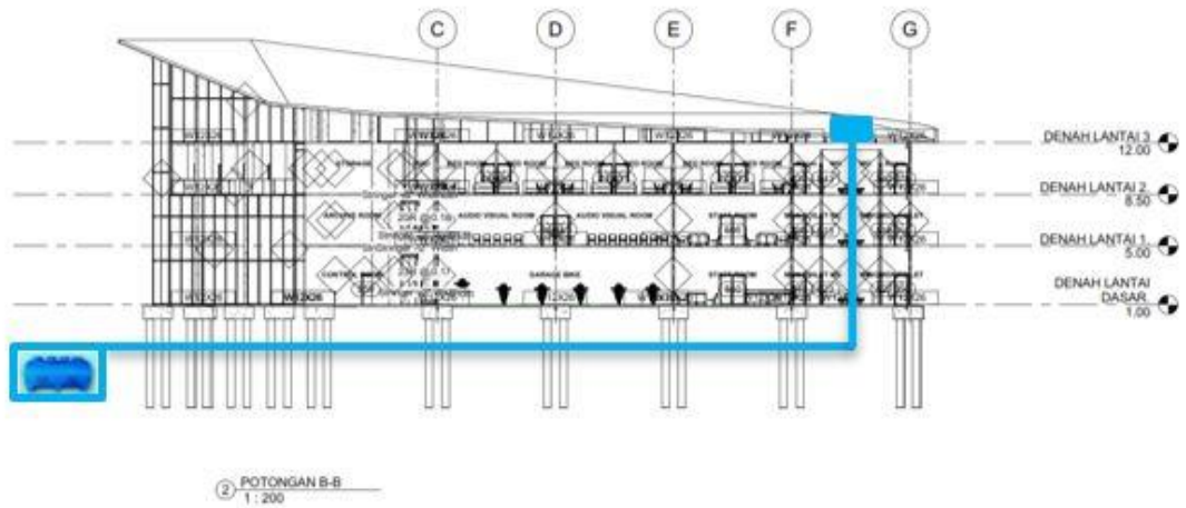
Gambar 6. 27 Utilitas Air Bersih 2
