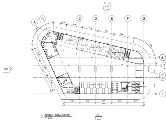
Gambar 6. 8 Denah Sekolah Balap Lantai 1
