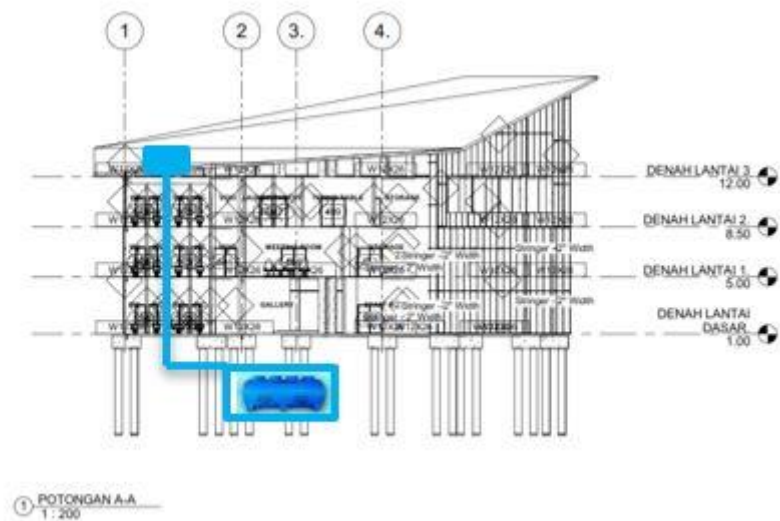
Gambar 6. 25 Utilitas Air Bersih
