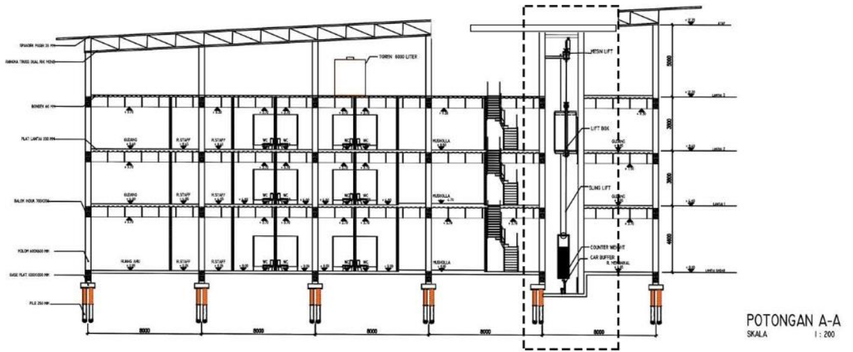
Gambar 6. 12 Potongan A-A
