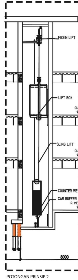
Gambar 6. 23 Potongan Prinsip 2
