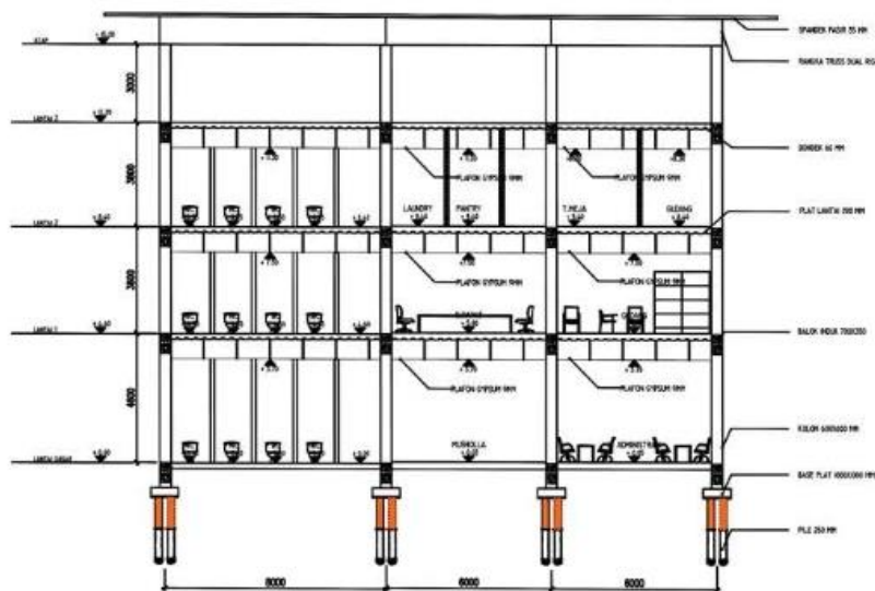
Gambar 6. 9 Potongan B-B
