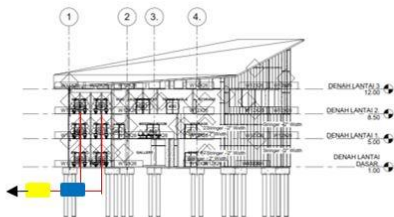
Gambar 6. 28 Utilitas Air Kotor 2
