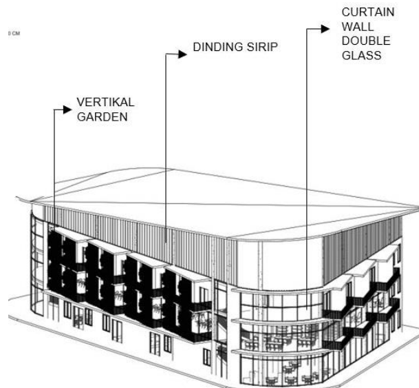
Gambar 6. 20 Sistem Konstruksi
