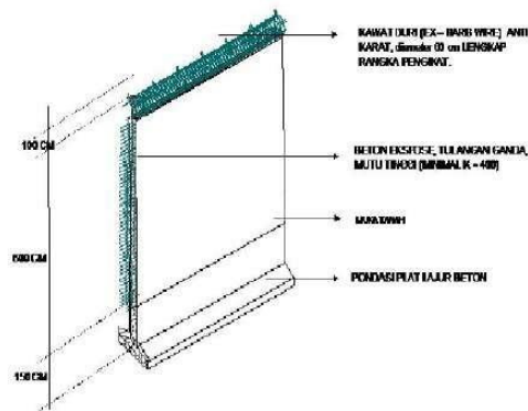
Gambar 2. 2 Pagar Keliling dalam
