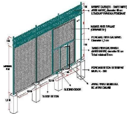
Gambar 2. 1 Pagar Pembatas sisi luar
