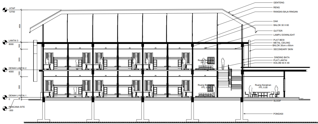
Gambar 6. 11 Potongan Bangunan 1
