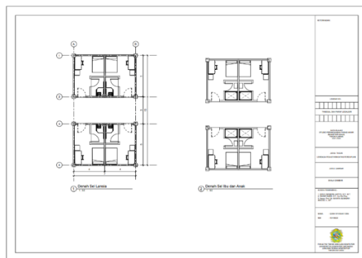
Gambar 6. 6 Denah Lansia dan Ibu&Anak
