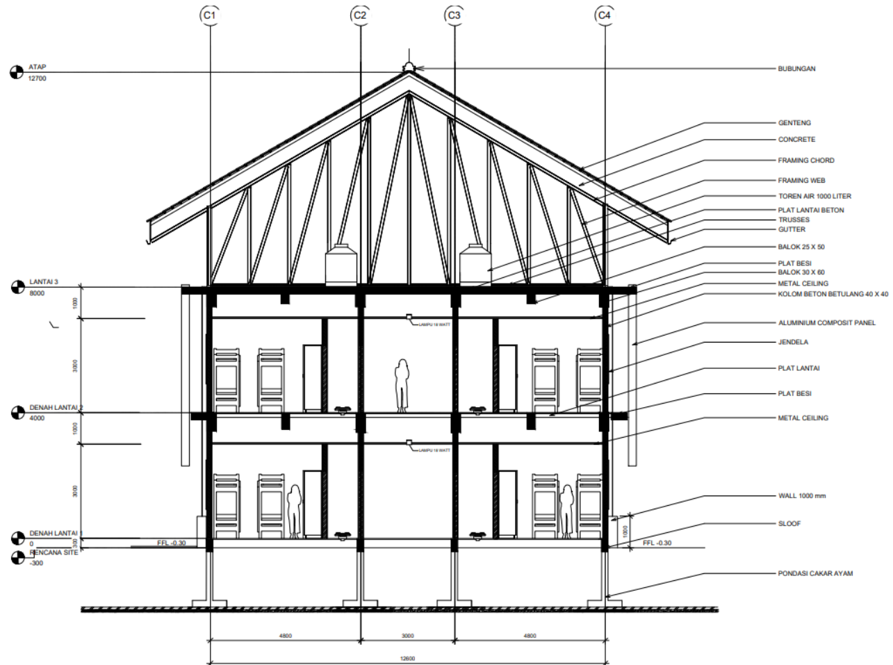
Gambar 6. 10 Potongan Bangunan 2
