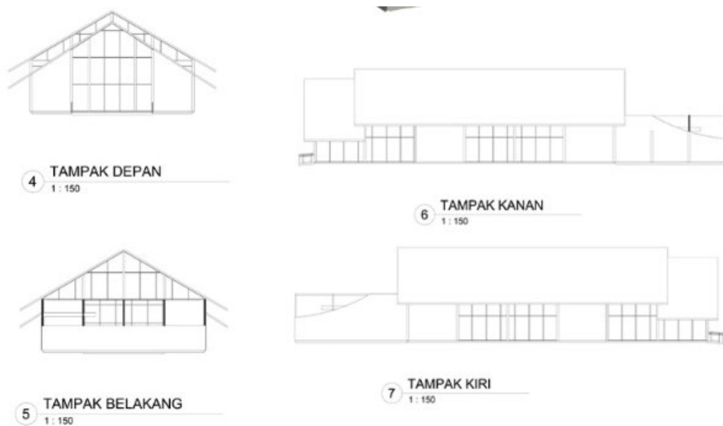
Gambar 6. 21 Tampak Bangunan Penerimaan Sumber : Dokumen Pribadi
