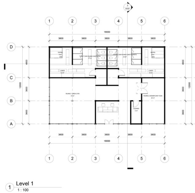
Gambar 6. 8 Denah Gym Centre Sumber : Dokumen Pribadi
