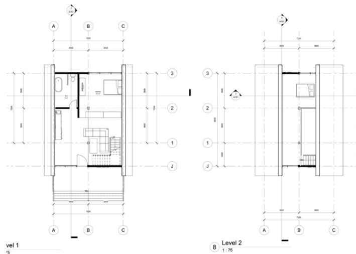
Gambar 6. 6 Denah Cottage Presidential Sumber : Dokumen Pribadi
