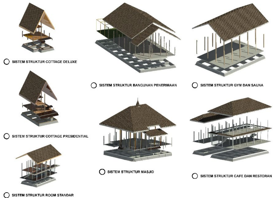
Gambar 6. 25 Sistem Struktur Sumber Dokumen Pribadi
