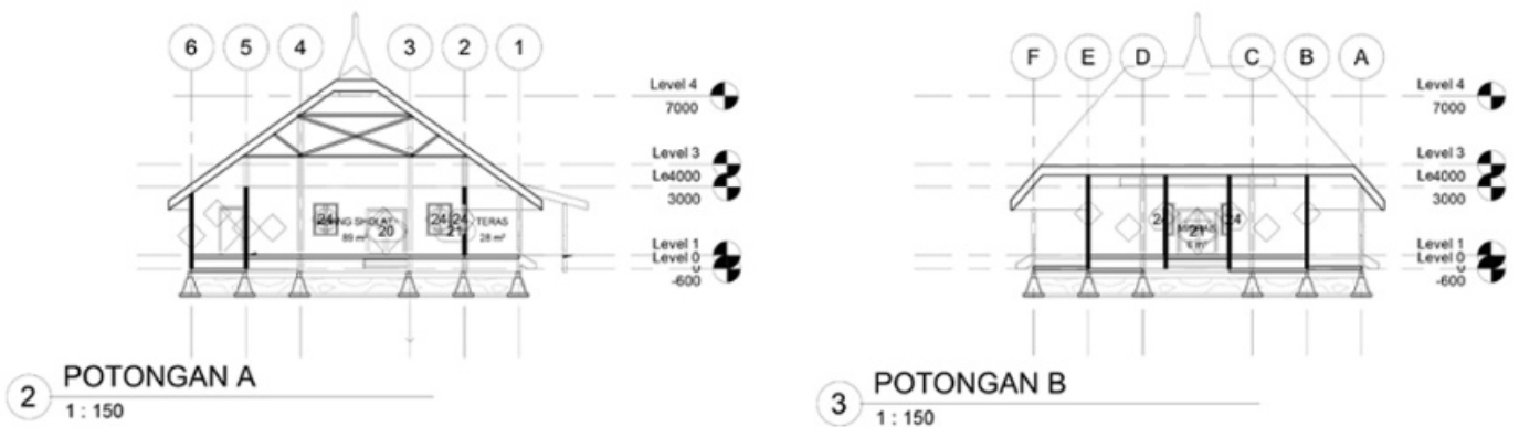
Gambar 6. 17 Potongan Mushola Sumber : Dokumen Pribadi
