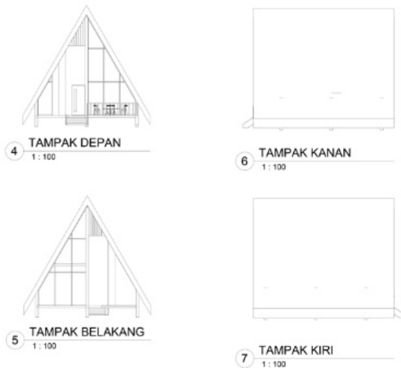
Gambar 6. 19 Tampak Cottage Deluxe Sumber : Dokumen Pribadi
