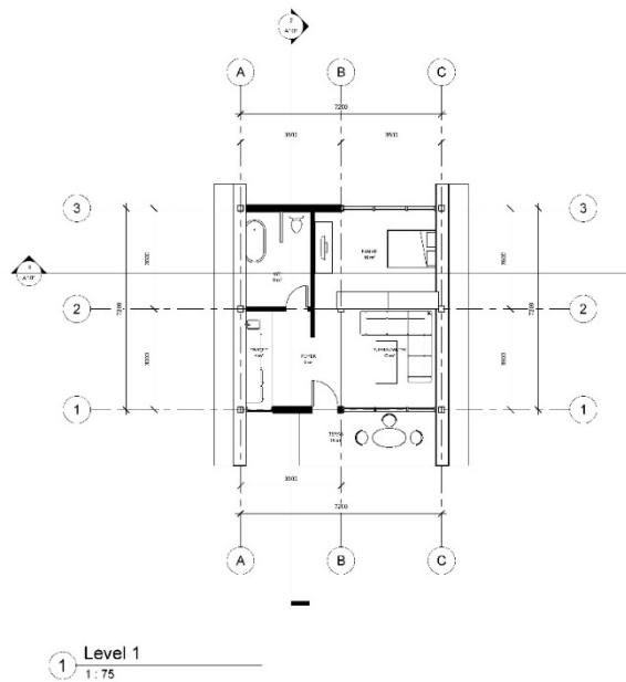
Gambar 6. 5 Denah Cottage Deluxe Sumber : Dokumen Pribadi
