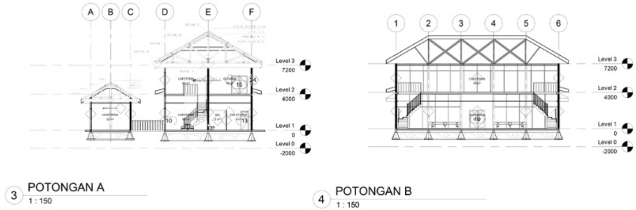
Gambar 6. 16 Potongan Cafe dan Restoran Sumber : Dokumen Pribadi
