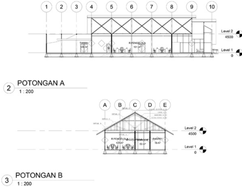
Gambar 6. 14 Potongan Bangunan Penerimaan Sumbe : Dokumen Pribadi
