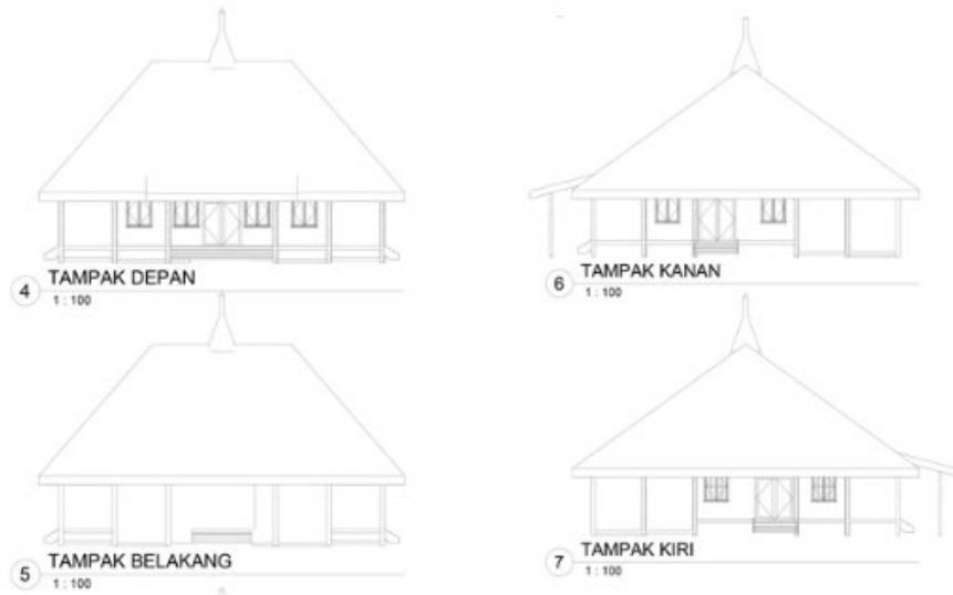
Gambar 6. 24 Tampak Mushola Sumber : Dokumen Pribadi
