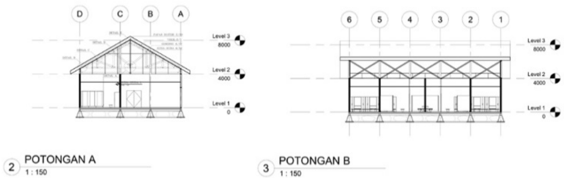
Gambar 6. 15 Potongan Gym Centre Sumber : Dokumen Pribadi
