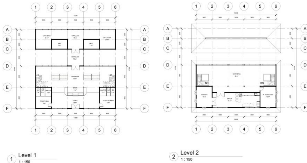
Gambar 6. 9 Denah Cafe dan Restoran Sumber : Dokumentasi Pribadi
