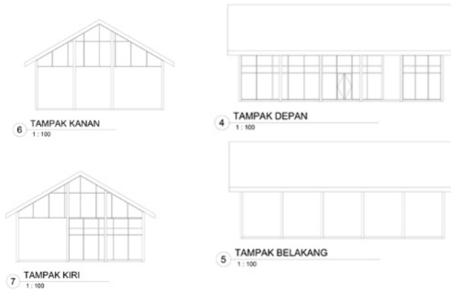
Gambar 6. 22 Tampak Gym Centre Sumber : Dokumen Pribadi
