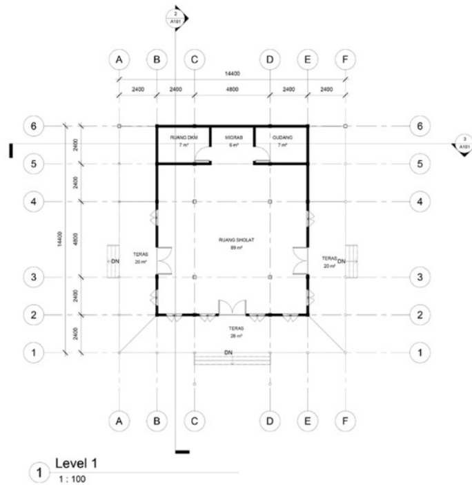
Gambar 6. 10 Denah Mushola Sumber : Dokumen Pribadi
