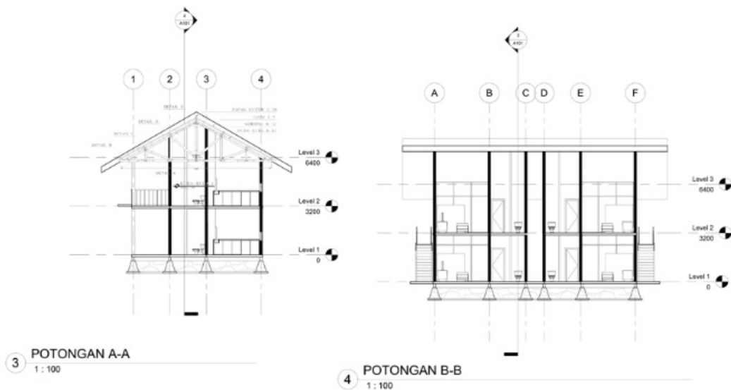
Gambar 6. 11 Potongan Cottage Standar Room Sumber : Dokumen Pribadi
