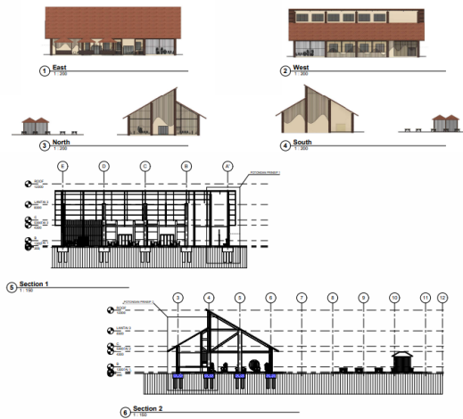
Gambar 42. Tampak Dan Potongan Cafe
