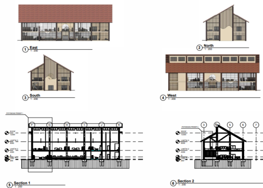
Gambar 44. Tampak Dan Potongan Coworking 1
