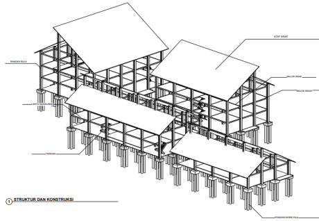
Gambar 48. Sistem Struktur
