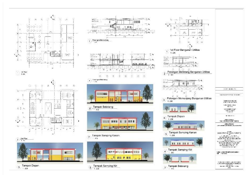
Gambar 6.11 DTP Bangunan Pengelola dan Servis Sumber: Dokumen Pribadi (2022)
