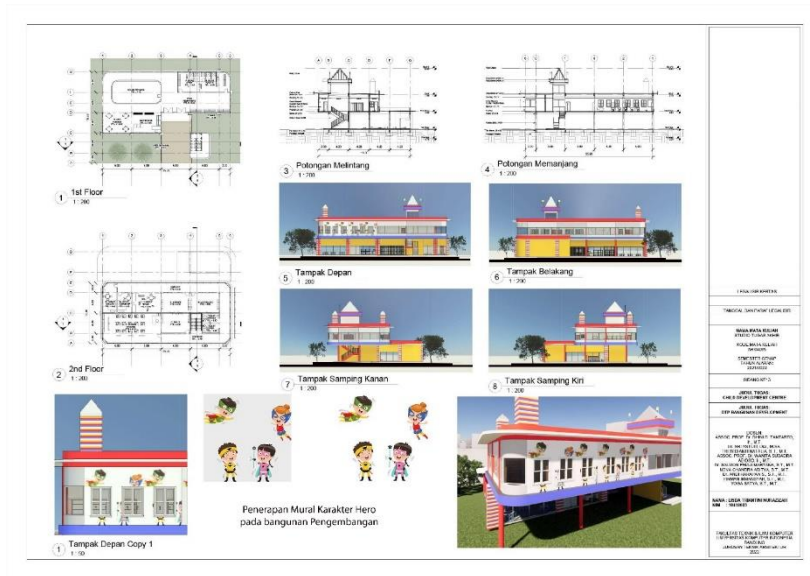
Gambar 6.9 DTP Bangunan Pengembangan Sumber: Dokumen Pribadi (2022)
