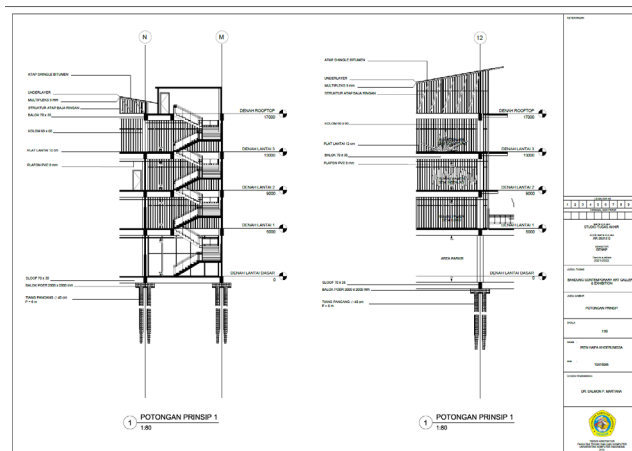
Gambar 6. 16 Potongan Prinsip Sumber: Dokumen Pribadi
