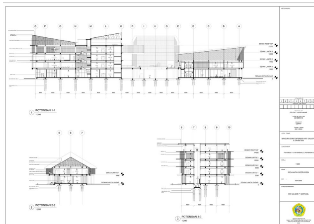
Gambar 6. 8 Potongan 1, Potongan 2, Potongan 3
