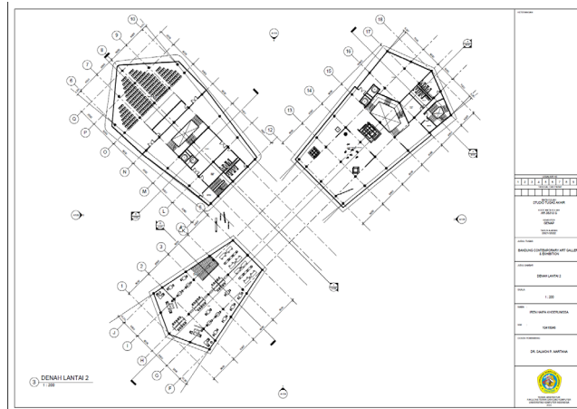
Gambar 6. 5 Denah Lantai 2 Sumber: Dokumen Pribadi
