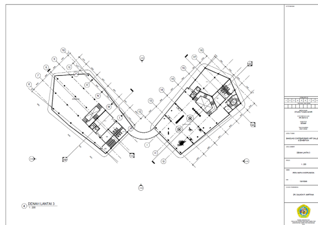
Gambar 6. 6 Denah Lantai 3 Sumber: Dokumen Pribadi
