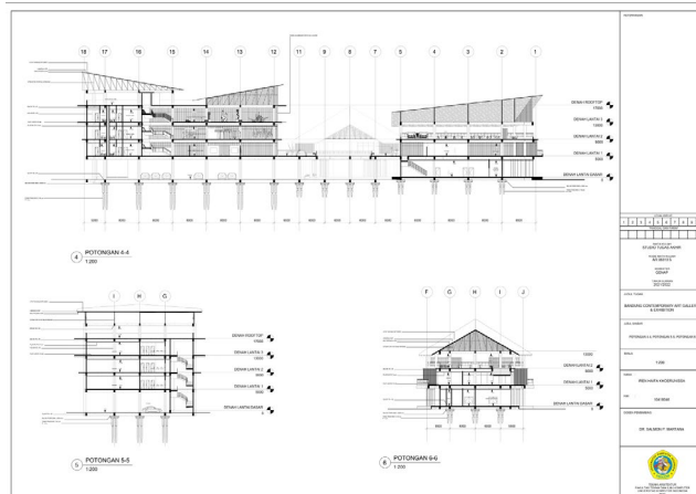
Gambar 6. 9 Potongan 4, Potongan 5, Potongan 6 Sumber: Dokumen Pribadi
