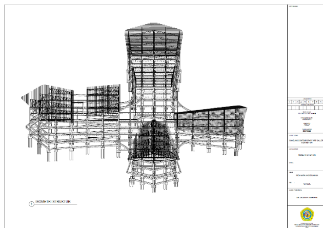
Gambar 6. 12 Isometri Struktur
