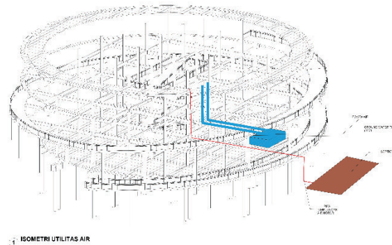
Gambar 6. 16 Isometri Utilitas Air Bersih dan Air Kotor
