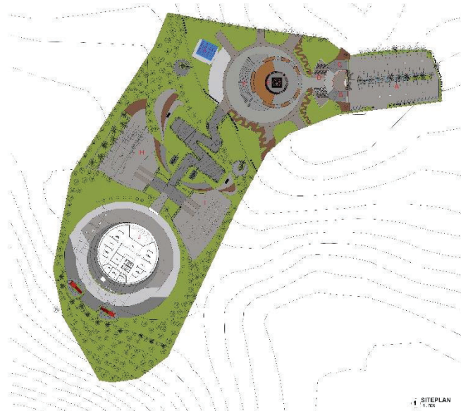
Gambar 6. 2 Siteplan
