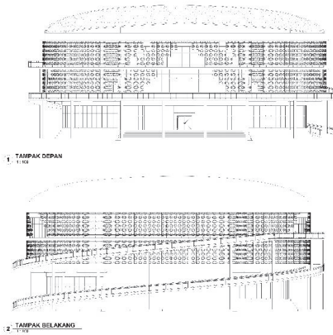
Gambar 6. 10 Tampak depan belakang Museum
