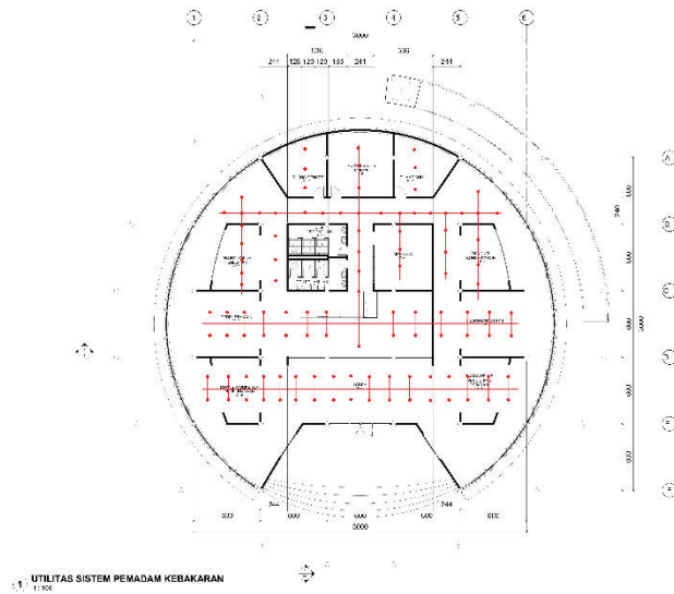
Gambar 6. 17 Instalasi Penanggulangan Kebakaran
