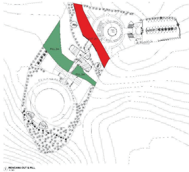
Gambar 6. 3 Rencana Cut & Fill
