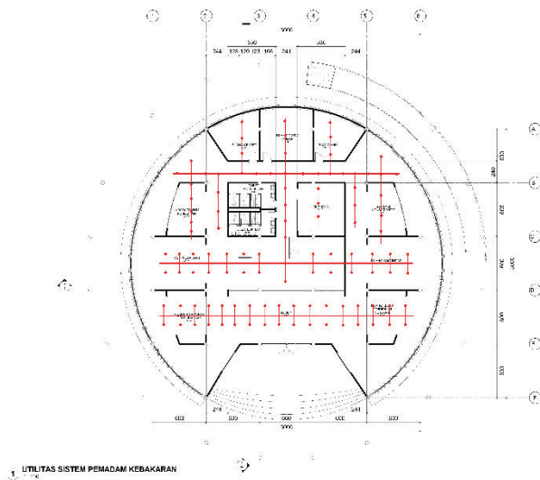
Gambar 6. 19 Instalasi Titik Sprinkler
