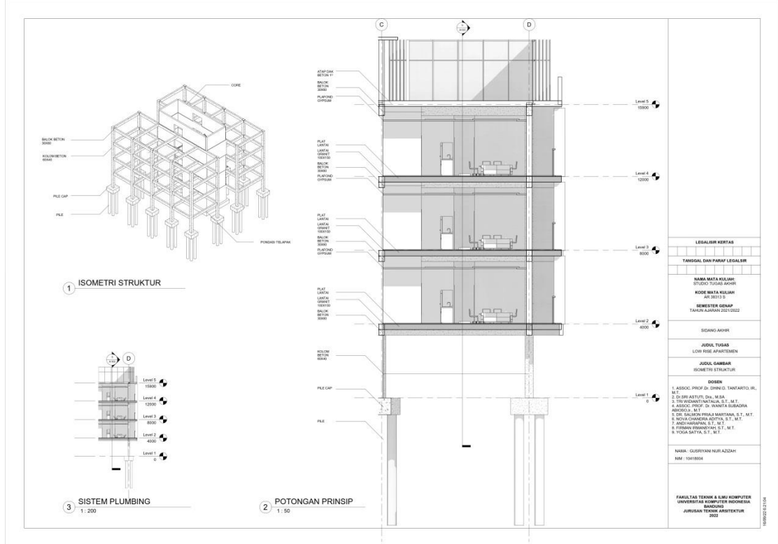
Gambar 6. 10 Isometri Struktur dan Potongan Prinsip Bangunan Apart Tipe 2
