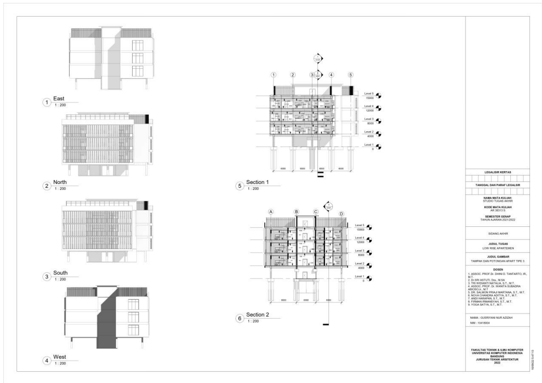
Gambar 6. 13 Tampak & Potongan Bangunan Apart Tipe 3
