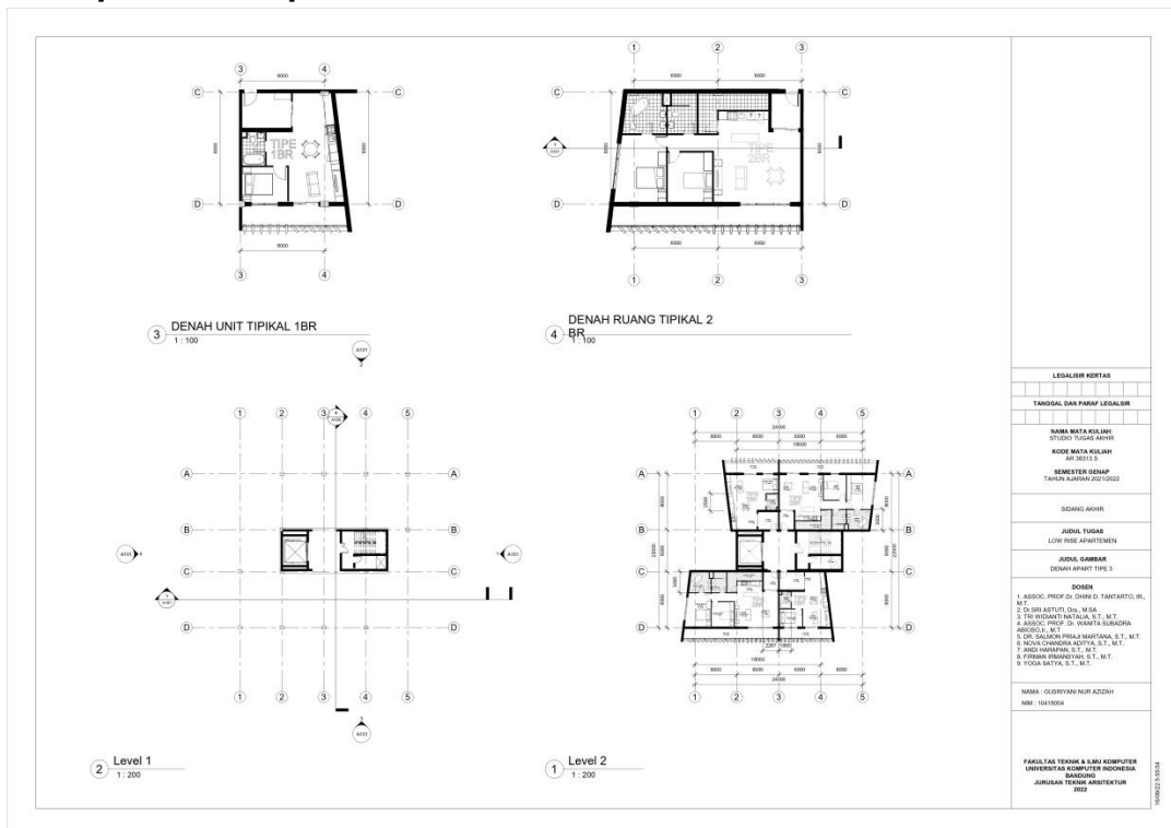
Gambar 6. 12 Denah Bangunan Apart Tipe 3
