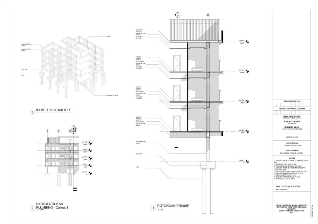
Gambar 6. 14 Isometri Struktur, Sistem Utilitas & Potongan Prinsip Bangunan Apart Tipe 3
