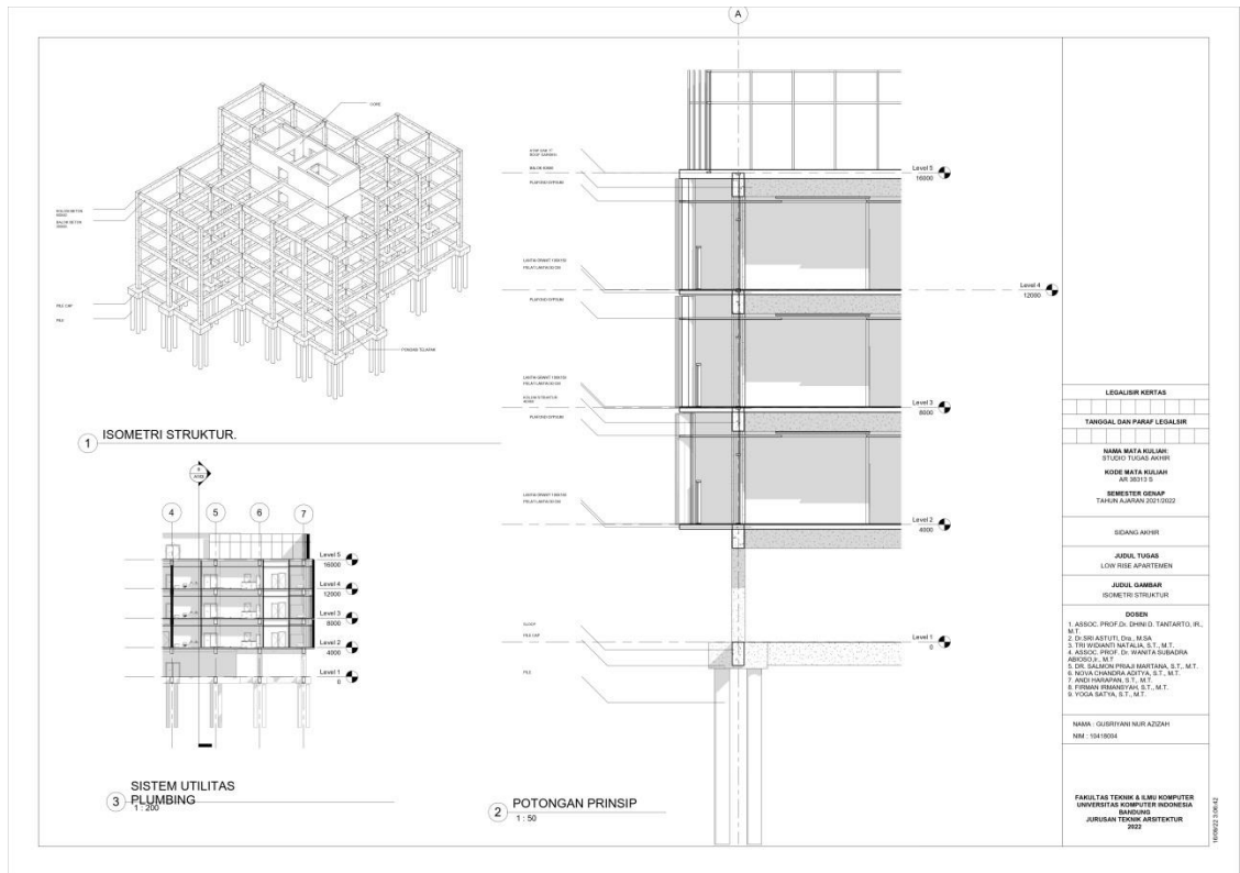
Gambar 6. 7 Isometri struktur, utilitas, dan potongan prinsip Bangunan Apart Tipe 1
