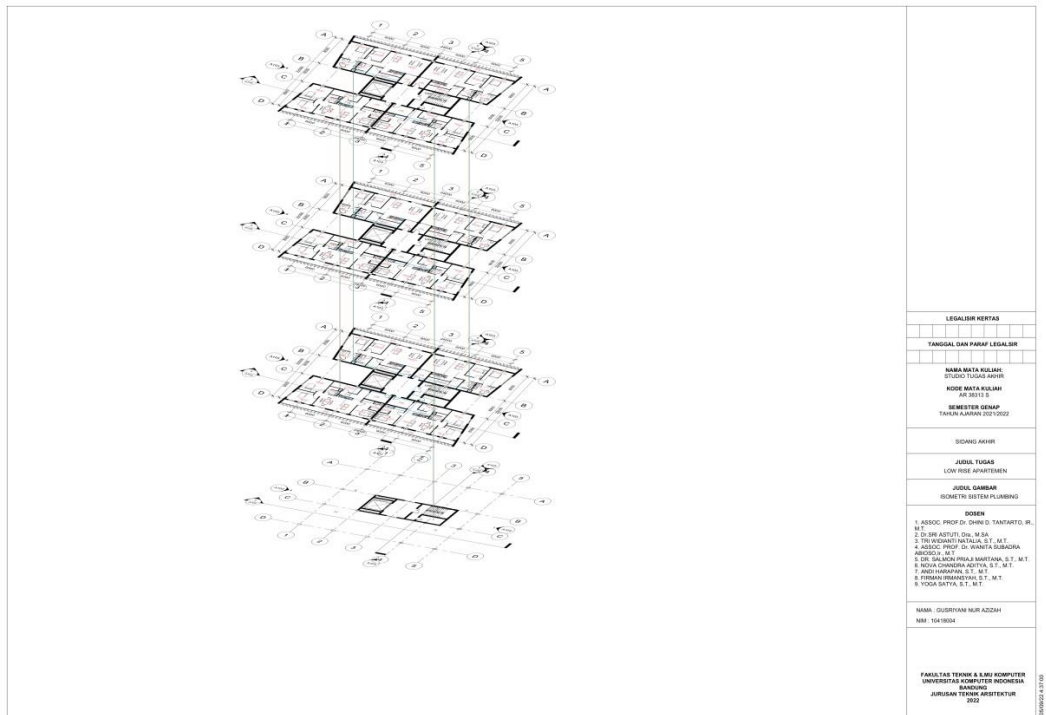
Gambar 6. 11 sistem utilitas Bangunan Apart Tipe 2
