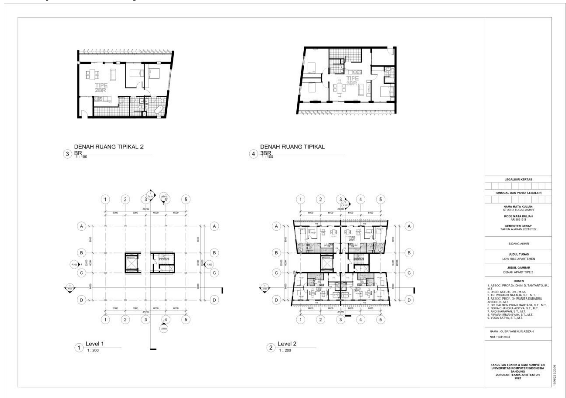
Gambar 6. 8 Denah Bangunan Apart Tipe 2
