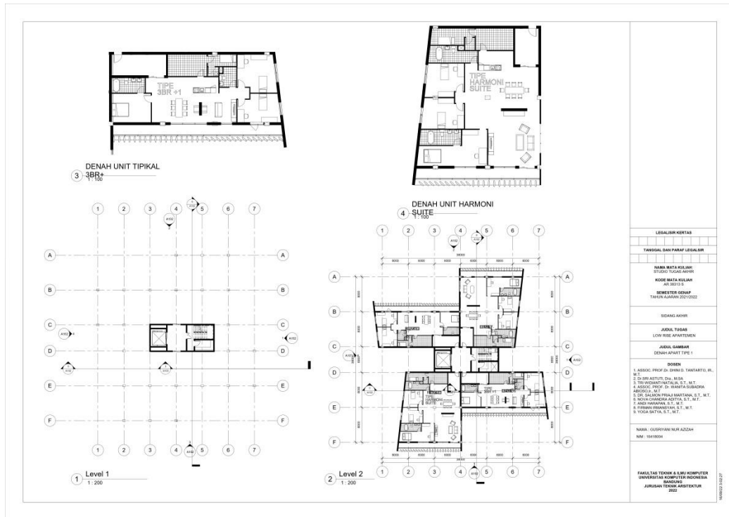
Gambar 6. 5 Denah Bangunan Apart Tipe 1
