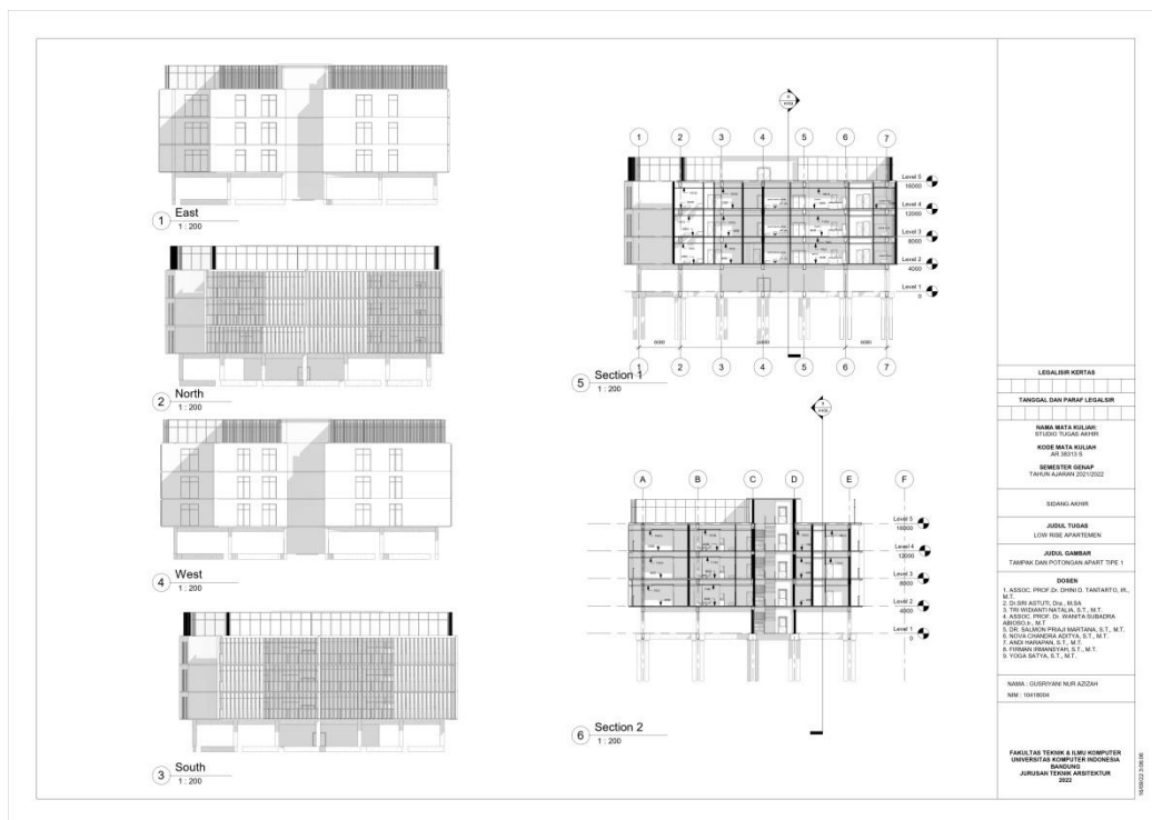
Gambar 6. 6 Tampak dan Potongan Bangunan Apart Tipe 1
