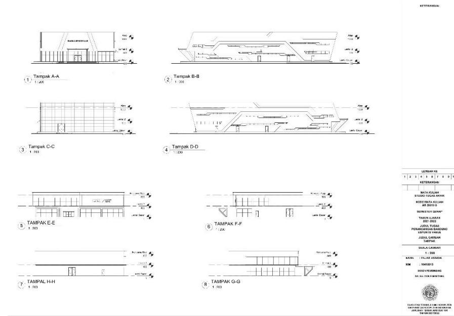
Gambar 6. 16 Tampak
