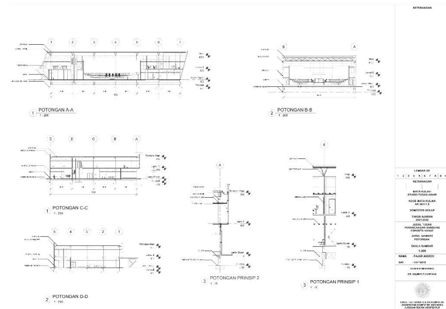
Gambar 6. 17 Potongan
