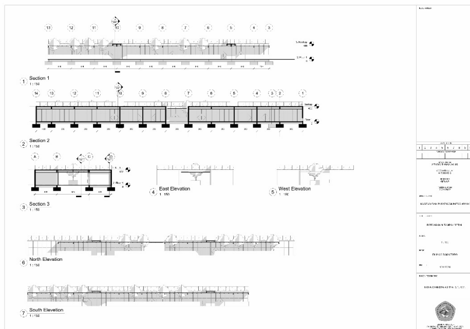
Gambar 6. 14 Tampak dan Potongan Retail
