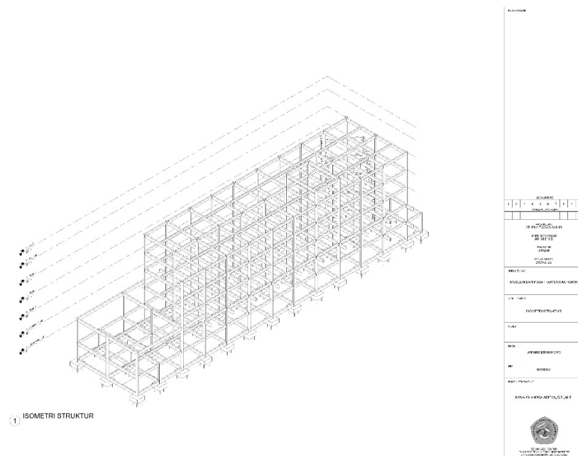
Gambar 6. 12 Isometri Sistem Struktur Sumber: Dokumentasi Pribadi, 2022
