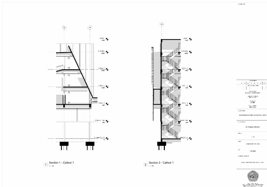
Gambar 6. 11 Potongan Prinsip Sumber: Dokumentasi Pribadi, 2022
