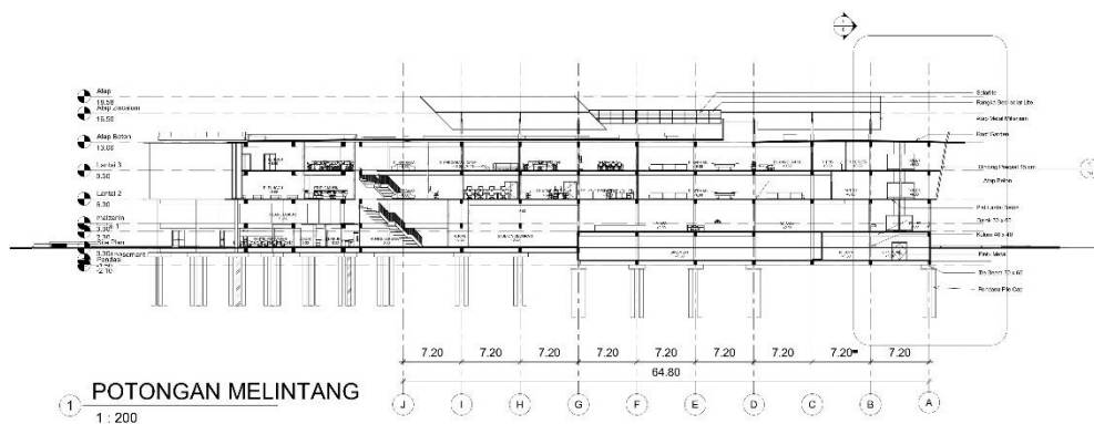
POTONGAN MELINTANG 1 : 200 Gambar 6. 7 Potongan Melintang Sumber: Dokumentasi Pribadi (2022)
