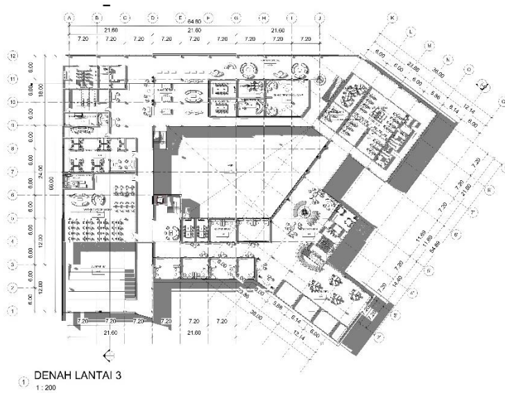
DENAH LANTAI 3 1 : 200 Gambar 6. 5 Denah Lantai Tiga Sumber: Dokumentasi Pribadi (2022)
