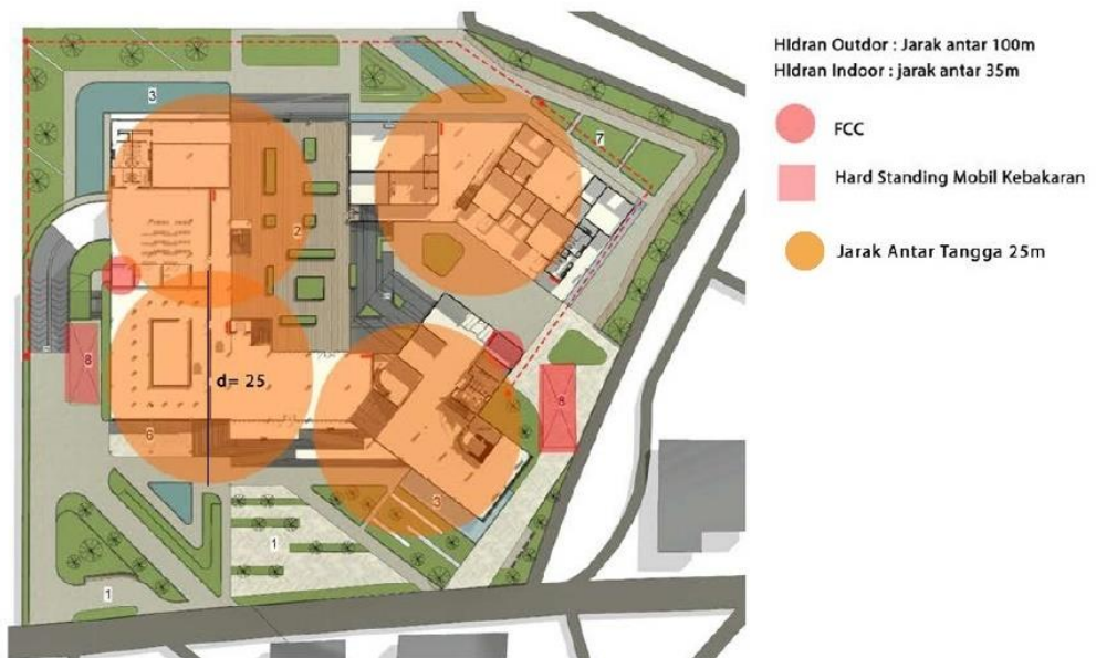
Gambar 6. 16 Utilitas Proteksi Kebakaran Sumber: Dokumentasi Pribadi (2022)
