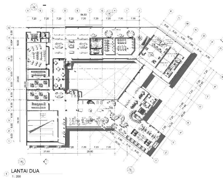
Gambar 6. 4 Denah Lantai Dua Sumber: Dokumentasi Pribadi (2022)
