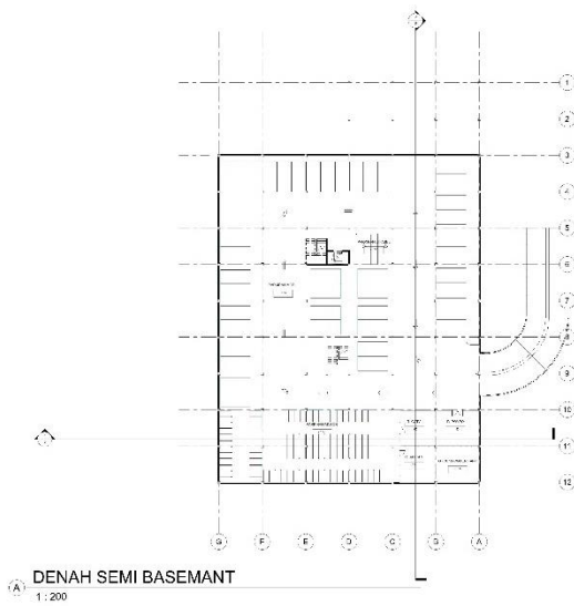
DENAH SEMI BASEMANT 1 : 200 Gambar 6. 6 Denah Semi Basement Sumber: Dokumentasi Pribadi (2022)
