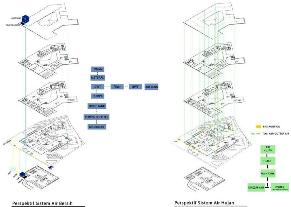
Gambar 6. 15 Perspektif Utilitas Air Bersih & Air Hujan Sumber: Dokumentasi Pribadi (2022)
