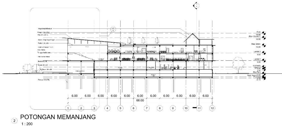
Gambar 6. 8 Potongan Memanjang Sumber: Dokumentasi Pribadi (2022)
