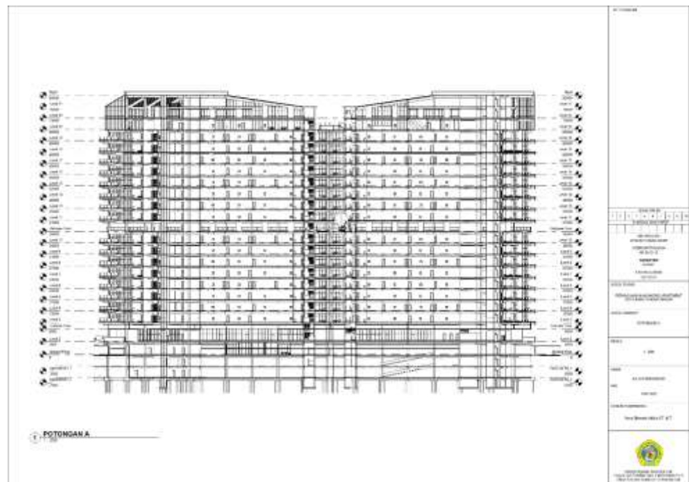
Gambar VI.10 Potongan A
