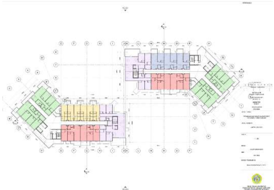
Gambar VI.7 Denah Lt. 6,10,15,19
