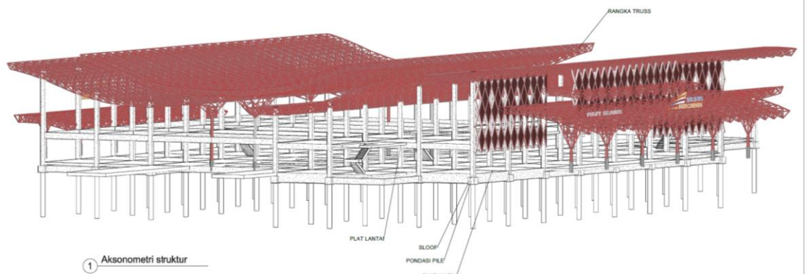
Gambar 6. 12 Aksonometri struktur
