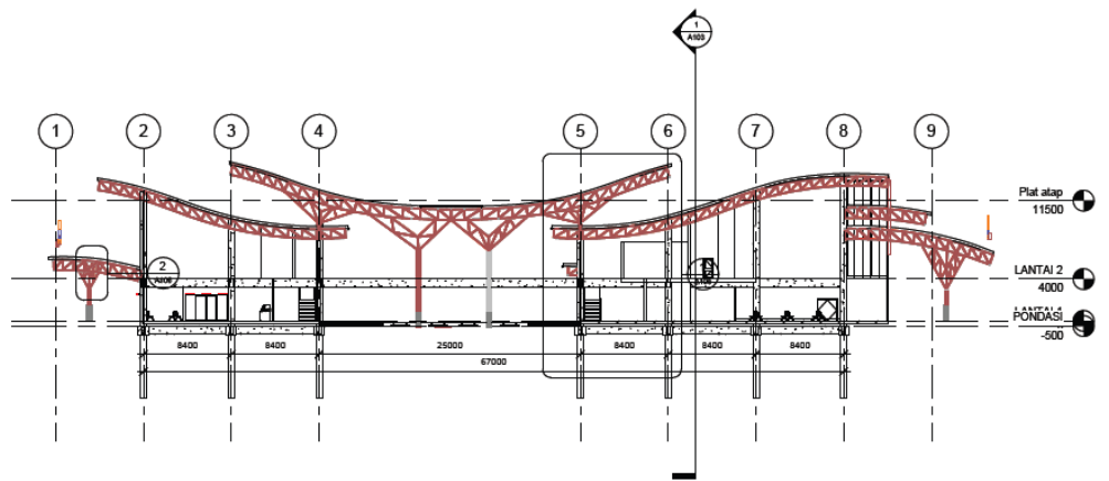
② Potongan Membujur 1 : 250
