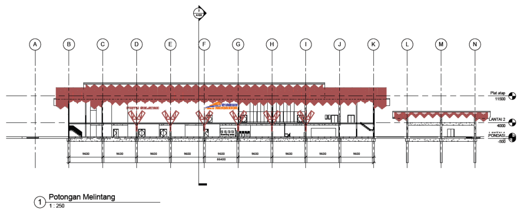
Gambar 6. 6 Potongan melintang
