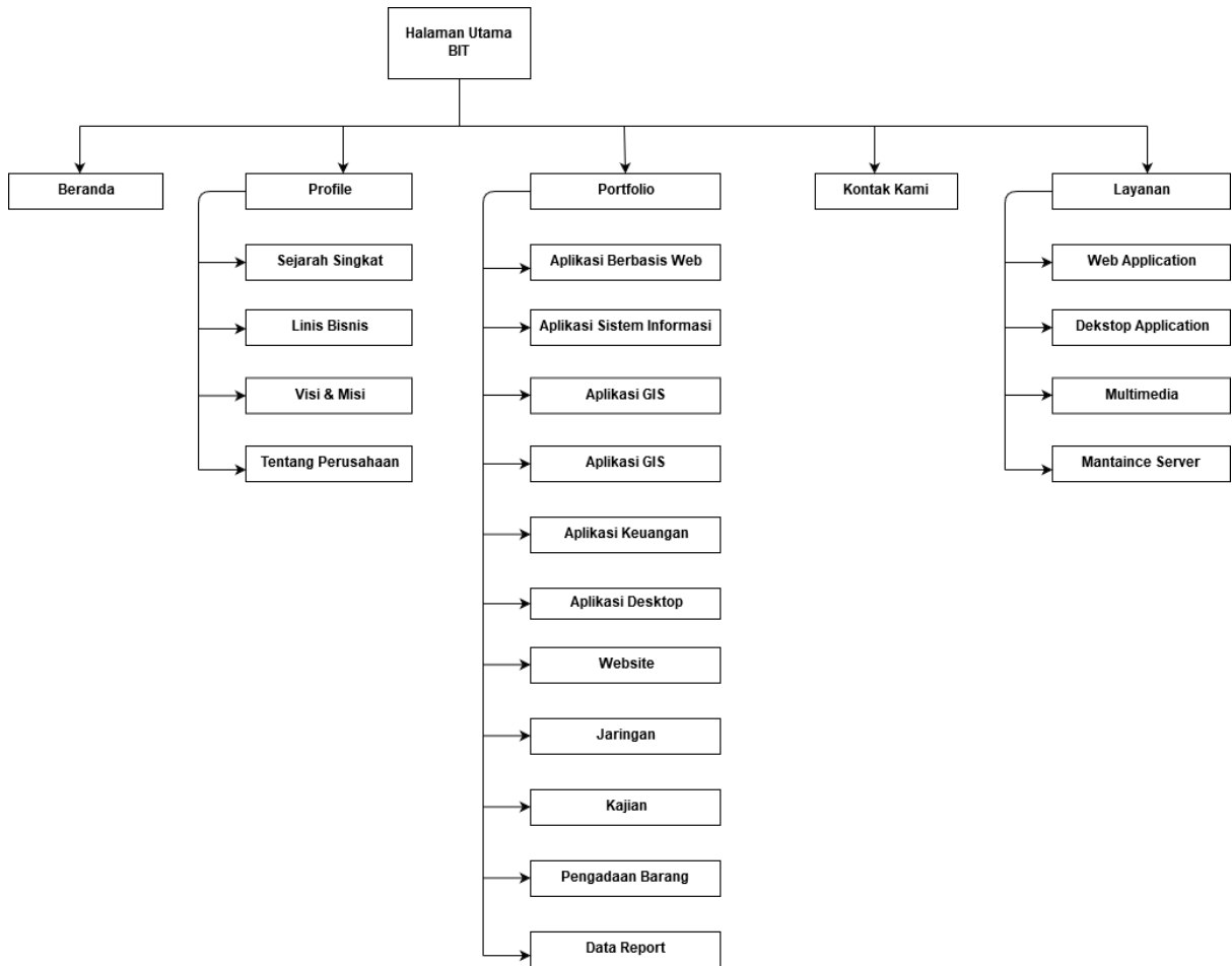
Gambar 0.12 Struktur Menu Sebelum Di Perbaharui
