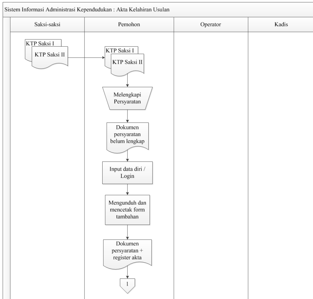
Gambar 4.2 : Flowmap yang diusulkan
