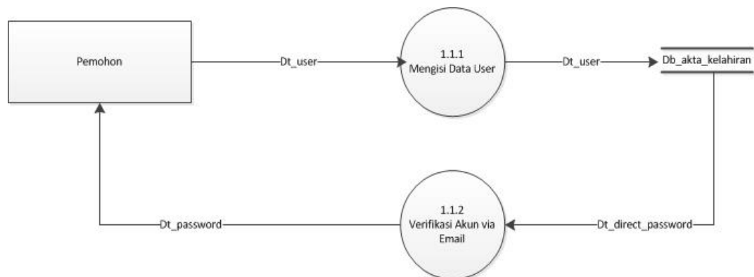
Gambar 4.10 : DFD Level 2 Proses 1.1 Pendaftaran Akun
