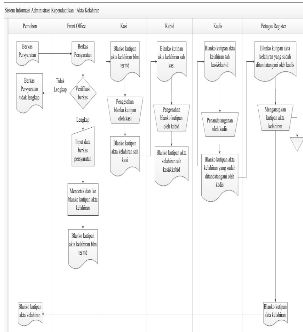
Gambar 4 1 : Flowmap sistem yang berjalan
