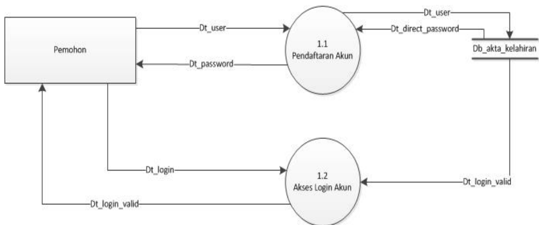
Gambar 4.8 : DFD Level 1 Proses 1 Login
