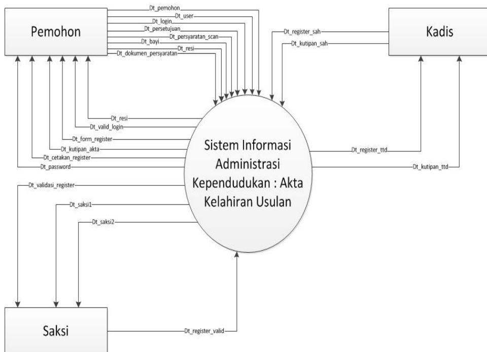
Gambar 4.6 : Diagram Konteks
