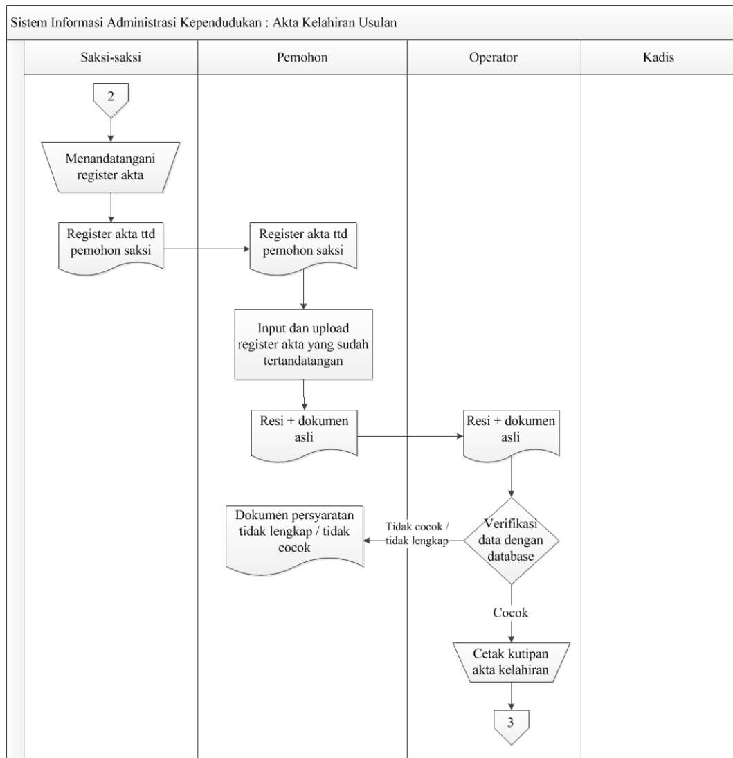
Gambar 4.4 : Flowmap yang diusulkan (lanjutan)
