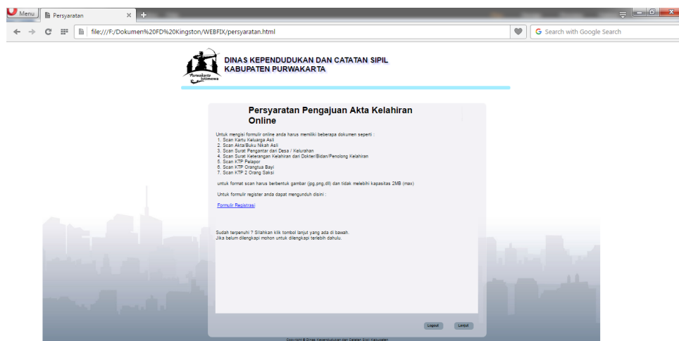
Gambar 4.16 : Halaman persyaratan
