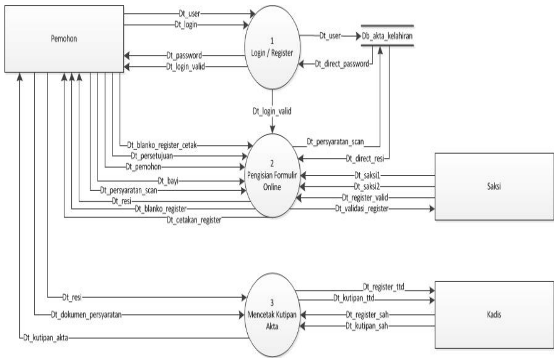
Gambar 4.7 : DFD Level 0
