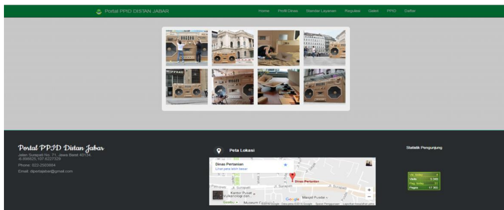
Gambar 4. 8. Menu Galeri
