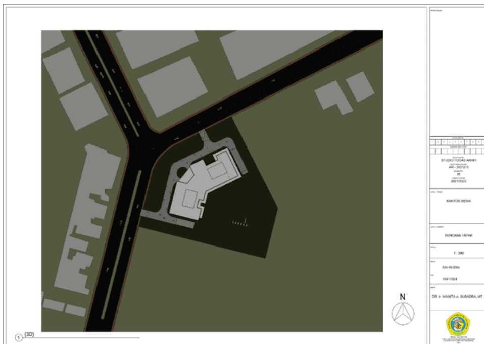
Gambar 6.2 1 Block Plan Sumber : Doc. Pribadi
