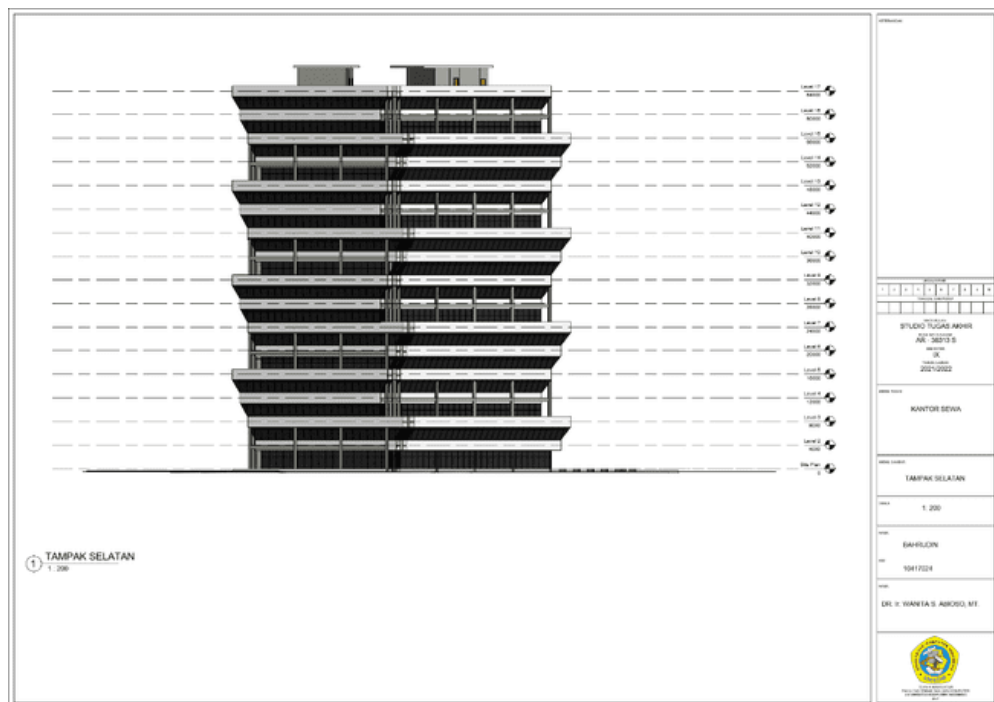
Gambar 6.2 13 Tampak Selatan Sumber : Doc. Pribadi
