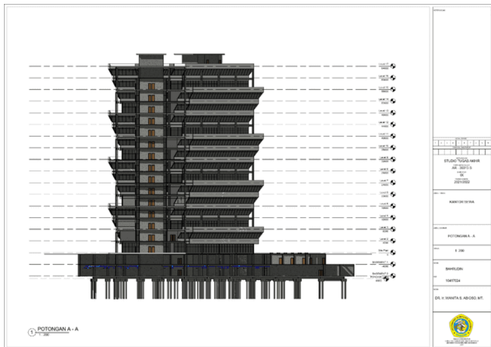
Gambar 6.2.9 Potongan A-A Sumber : Doc. Pribadi
