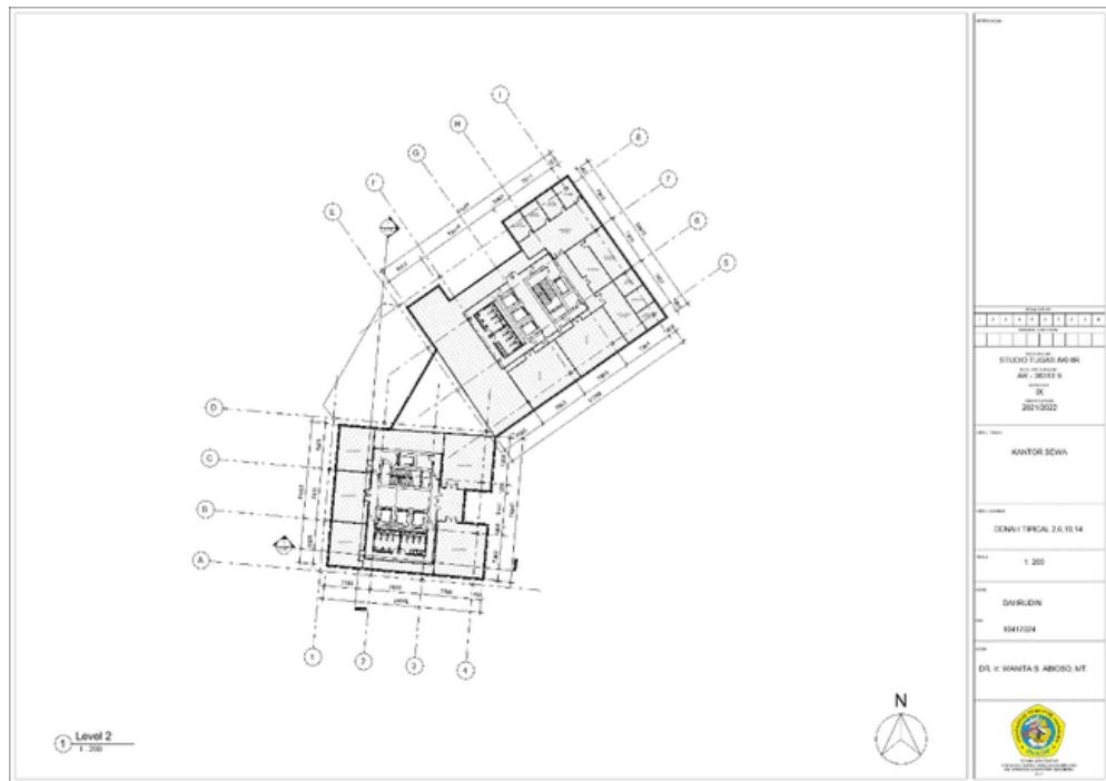
Gambar 6.2 4 Denah Lt. 2 Sumber : Doc. Pribadi
