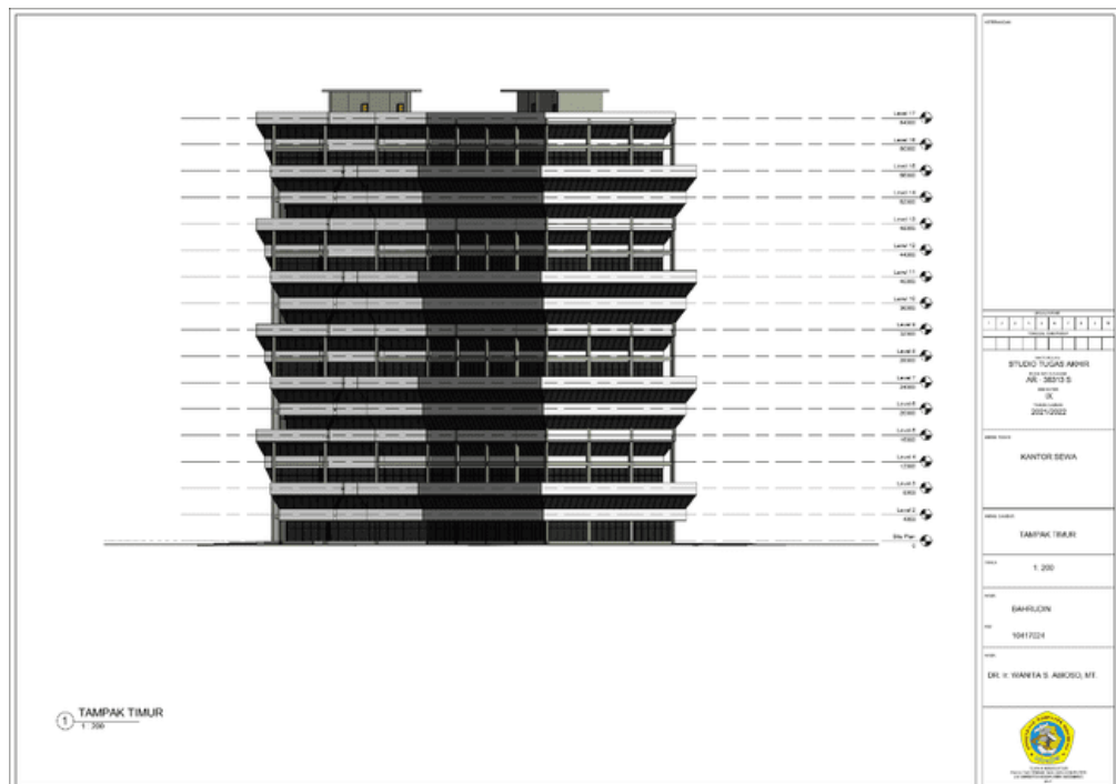
Gambar 6.2 11 Tampak Timur Sumber : Doc. Pribadi
