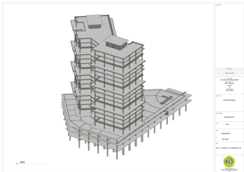
Gambar 6.2 17 Isometri Struktur Sumber : Doc. Pribadi
