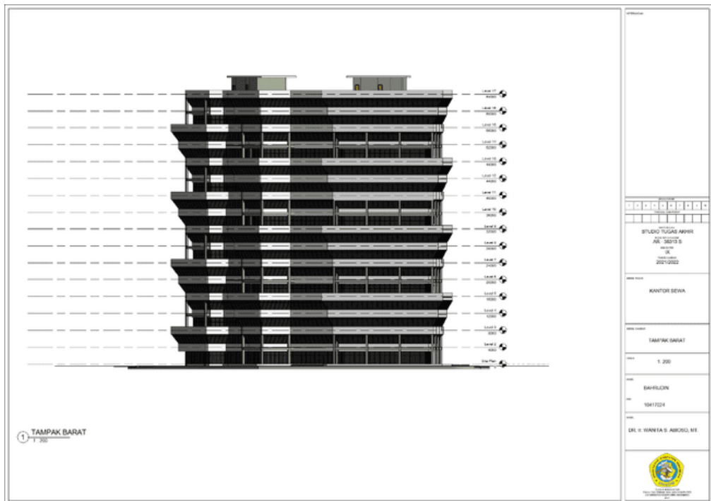
Gambar 6.2 14 Tampak Barat Sumber : Doc. Pribadi
