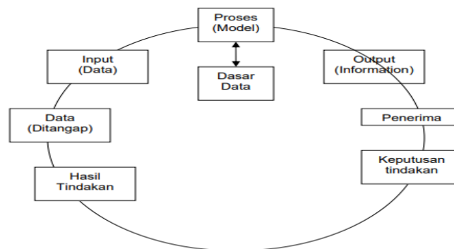
Gambar 2.3 1 Siklus Informasi
