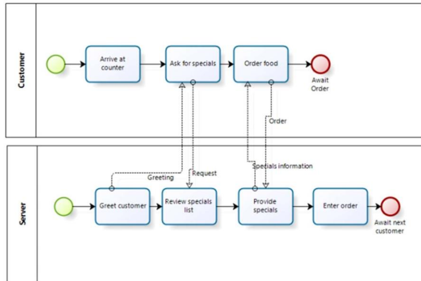
Gambar 2. 3 Contoh BPMN
