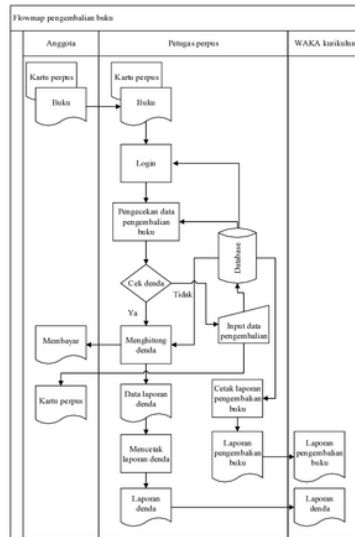
Gambar 6. Flowmap Pengembalian Buku Yang Diusulkan
