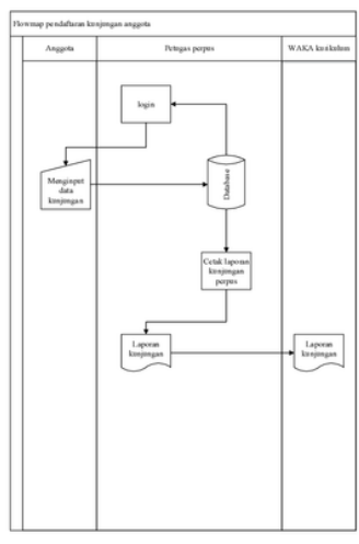
Gambar 3. Flowmap Pendaftaran Kunjungan Yang Diusulkan
