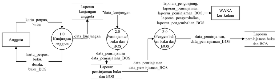
Gambar 2. DFD Level 1 Yang Diusulkan
