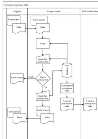
Gambar 4. Flowmap Peminjaman Buku Yang Diusulkan
