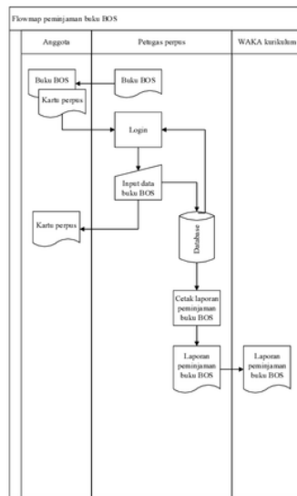
Gambar 5. Flowmap Peminjaman Buku BOS Yang Diusulkan
