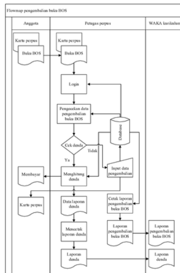
Gambar 7. Flowmap Pengembalian Buku BOS Yang Diusulkan
