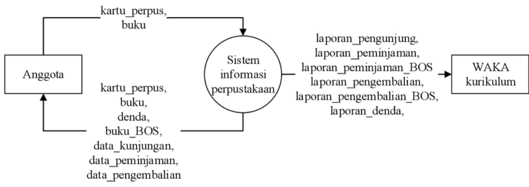
Gambar 1. Diagram Konteks Yang Diusulkan
